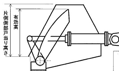
図－３ 起伏ゲート
