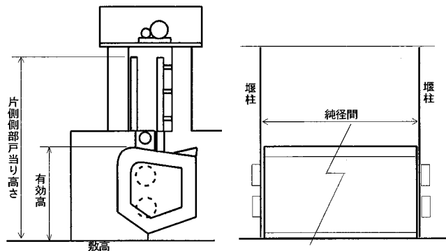
図－２ シェル構造ローラゲート
