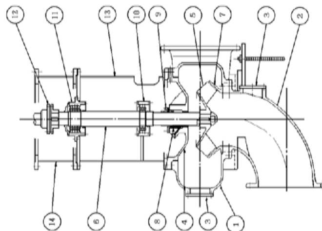
立軸渦巻斜戻ポンプ(1戻式)
