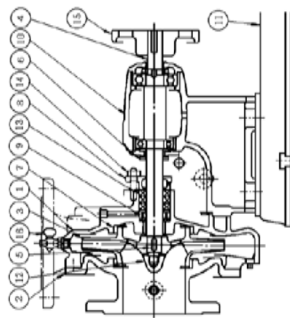
横軸片吸込車渦巻ポンプ
