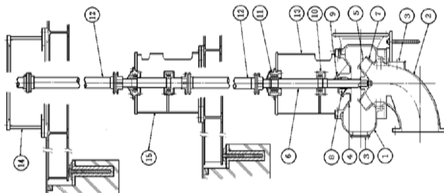
立軸渦巻斜戻ポンプ(多戻式)
