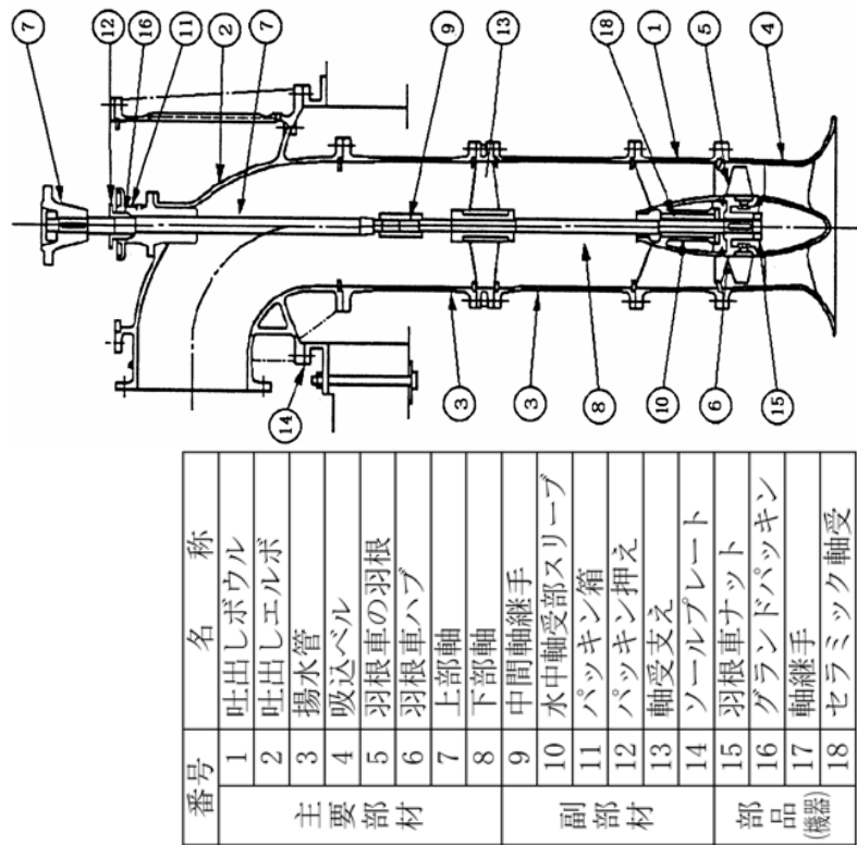
立式軸流ポンプ（一・二床式）
