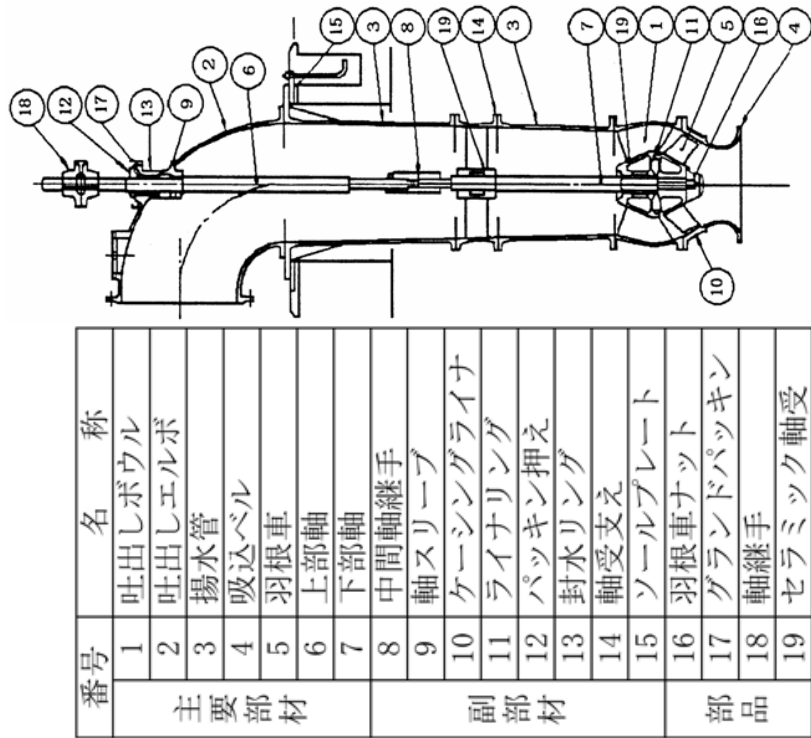
立式斜流ポンプ（一・二床式）
