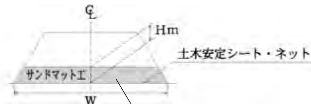
図 2-1 施工図
