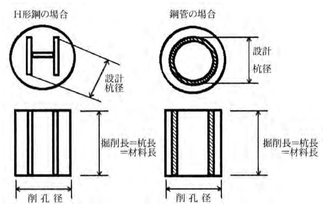
施工図
