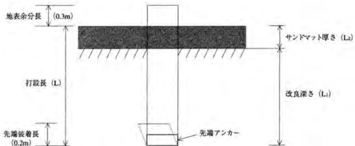
図 5.1 施工図
