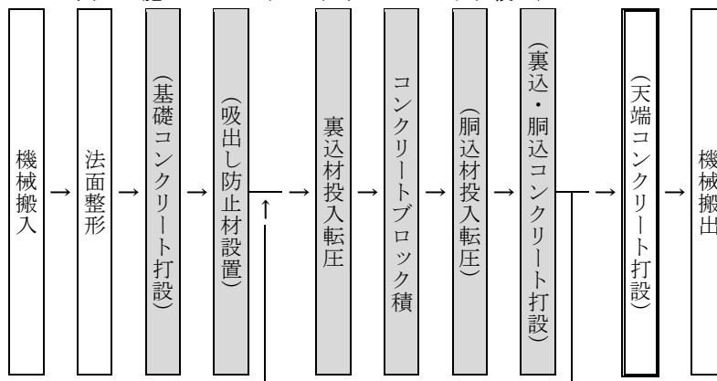
図 2-2 施工フロー（コンクリートブロック積工）
