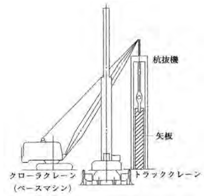
図 2-1 施工図
