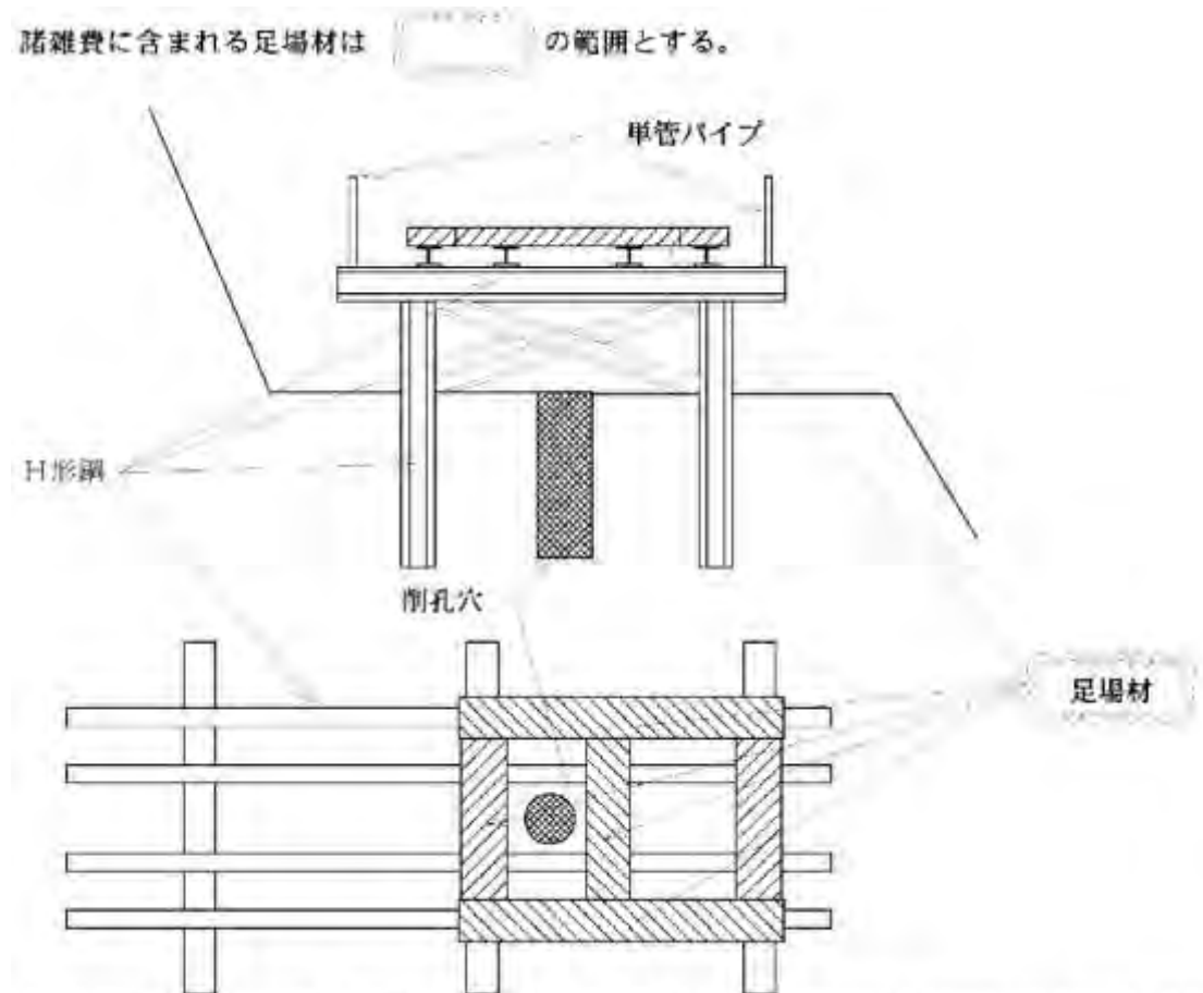
図 9-1 足場概念図
