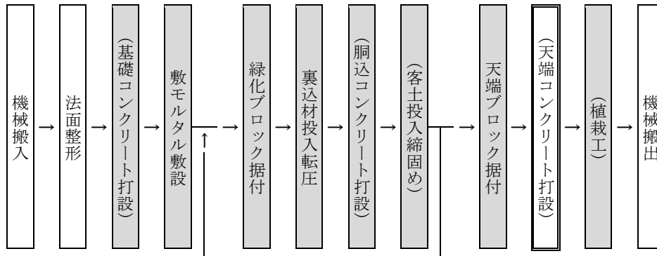
図 2-4 施工フロー（緑化ブロック積工）
