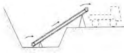
図 2.2 傾斜据付
