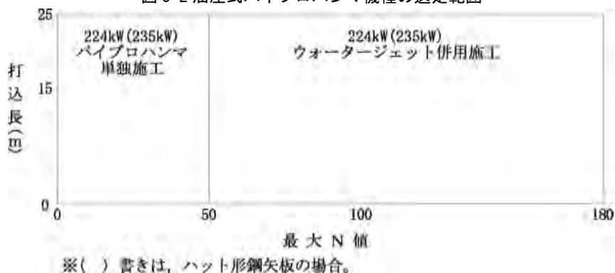
図 3-2 油圧式バイブロハンマ機種の選定範囲
