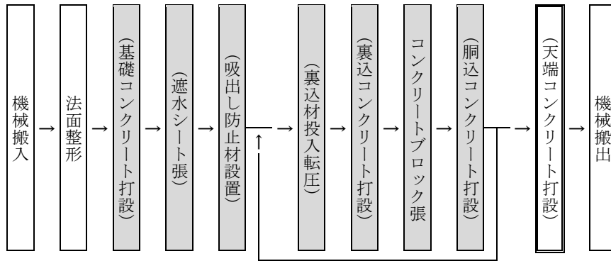
図 2-3 施工フロー（平ブロック張工，連節ブロック張工）
