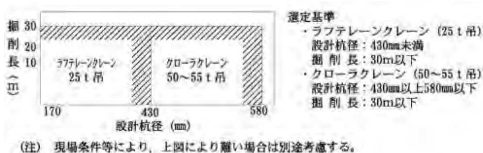
図 4-1 掘削用クレーン機種選定
