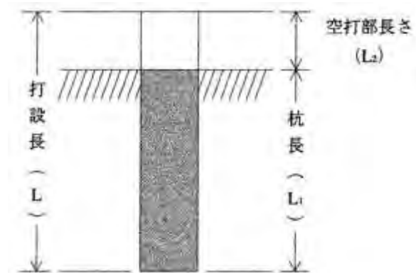
図 3-1 施工図
