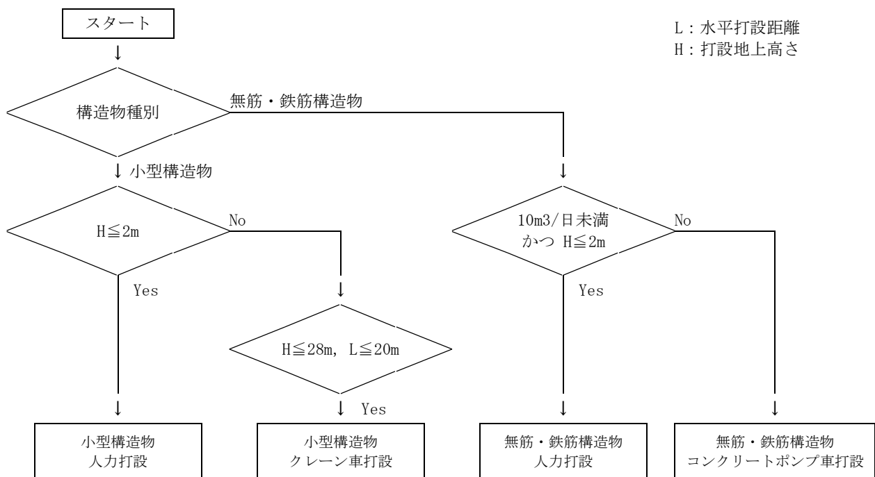
図 2.1 コンクリート打設工法の選定
