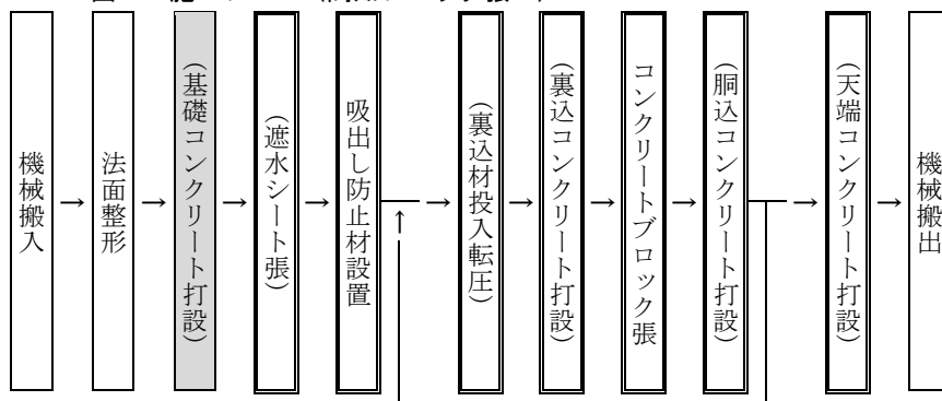
図 2-1 施工フロー（間知ブロック張工）
