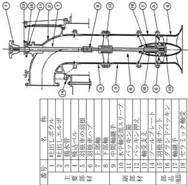
立軸軸流ポンプ（一・二床式）
