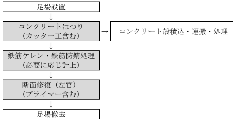
図 2-1 施工フロー
