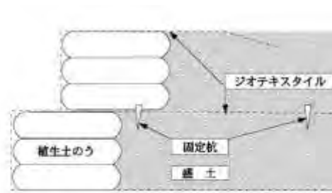
図B 巻込み工法(植生土のう)参考図
