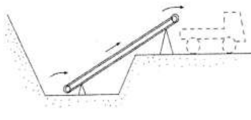
図 3. 2 傾斜据付
