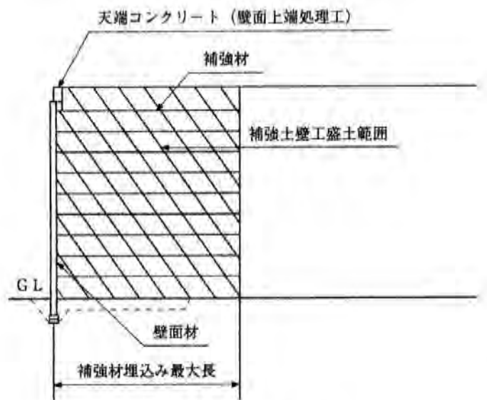
補強土壁工標準断面図
