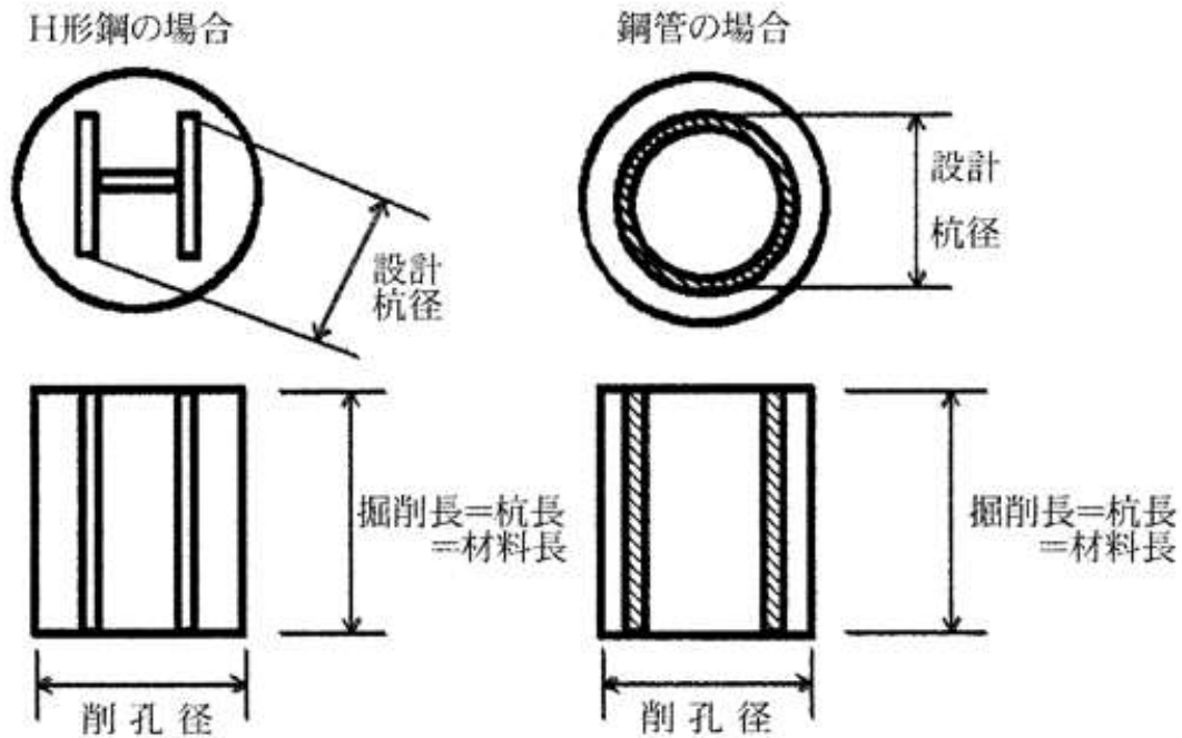
施工図
