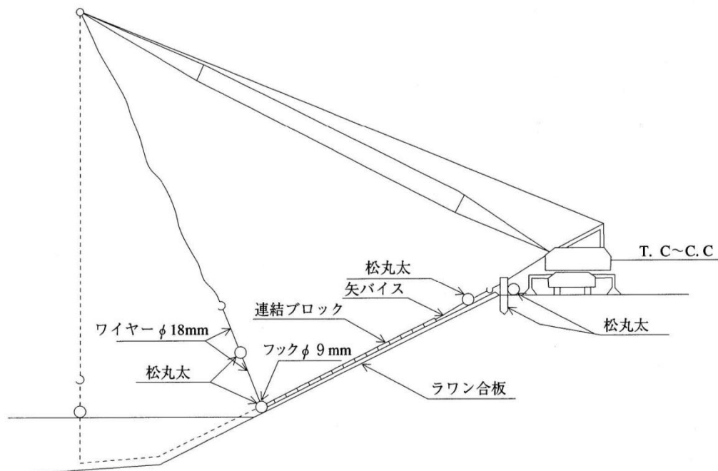
図 7-1 連節ブロック水中吊落し断面図
