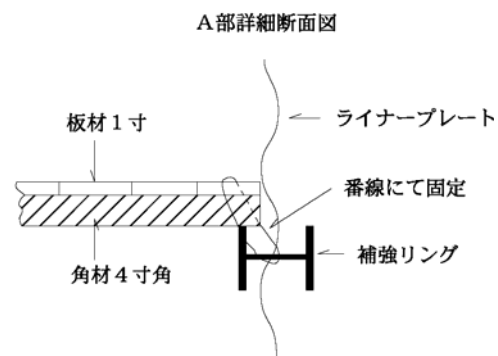
詳 細 図
