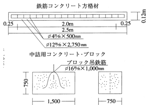
図 2-2 鉄筋コンクリート方絡材の標準図
