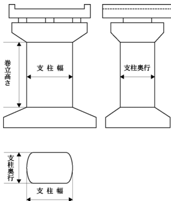
(1) 矩形（小判形を含む）支柱
