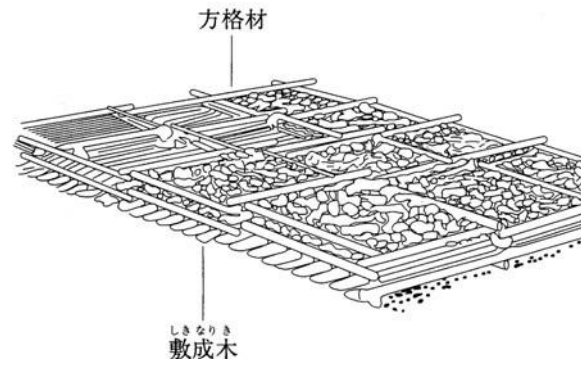
図 2-1 改良沈床工の概念図
