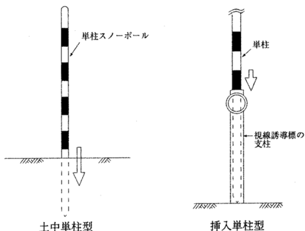
図 1-1 スノーポールの参考図
