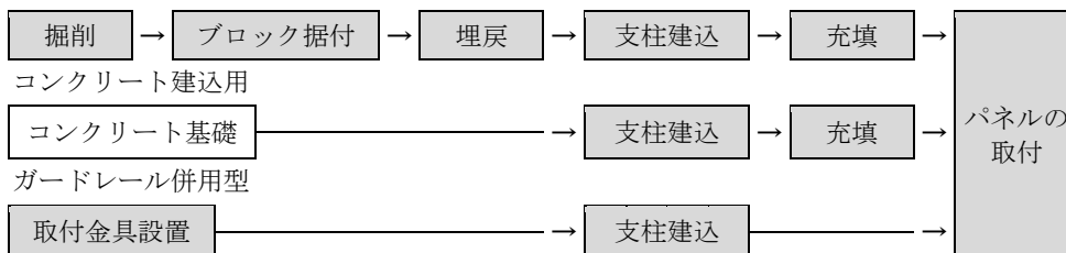
図 2-1 施工フロー
