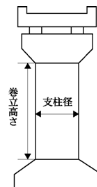
(2) 円形支柱
