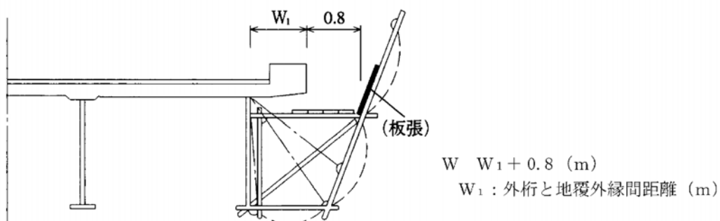
図-1 足場・防護標準図
