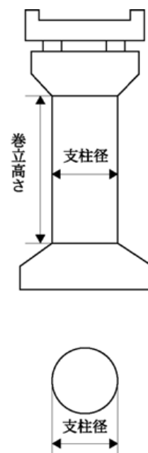
(2) 円形支柱
