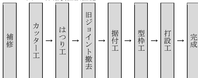
図-1 伸縮装置設置施工フロー
