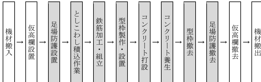
図 2-1 施工フロー
