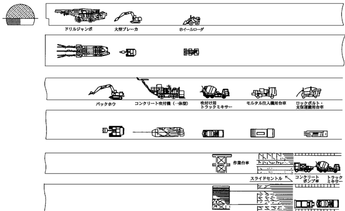
図 3.1 補助ベンチ付全断面工法
