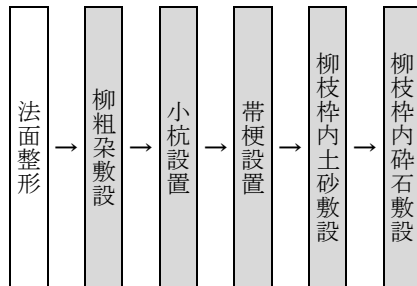
図 2-1 施工フロー（柳枝工）
