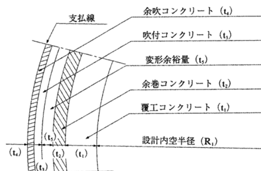
図 3.2 変形余裕を見込む場合
