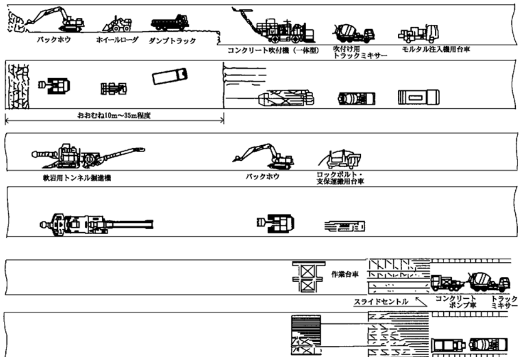
図 3.2 上半先進ベンチカット工法（上下半同時併進工法） 掘削機械配置例（2）（上半ずり出し作業時）
