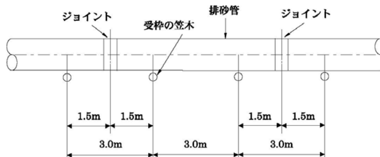
図 5-1 受枠の間隔
