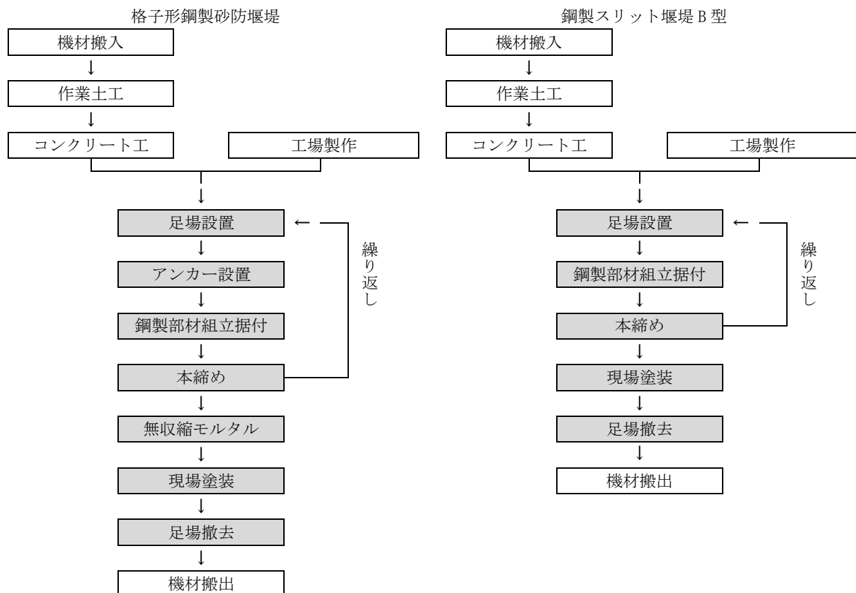
図 2-1 施工フロー
