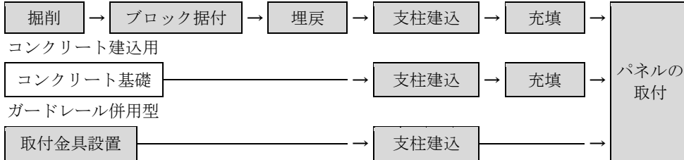
図 2-1 施工フロー
