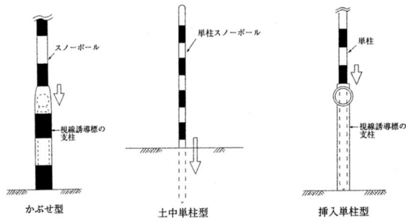
図 1.1 スノーポールの参考図
