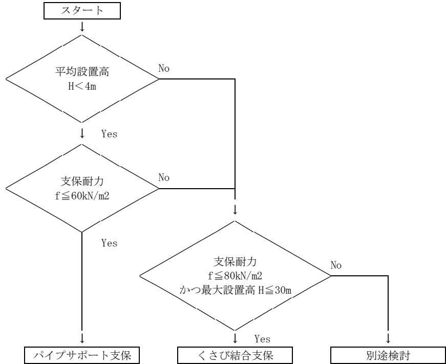
図 8-2 工法の選定
