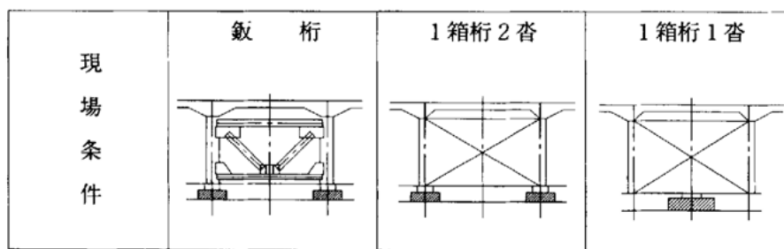
図 3.1 現場条件
