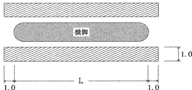
図 3.3 足場面積
