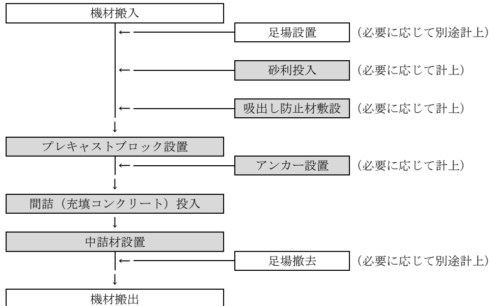
図 1-1 施工フロー
