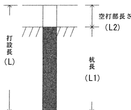
図 3.1 施工図
