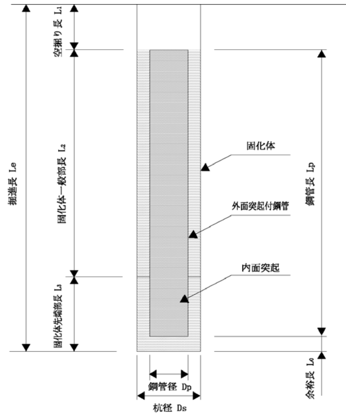
図 2.1 鋼管ソイルセメント杭のモデル図
