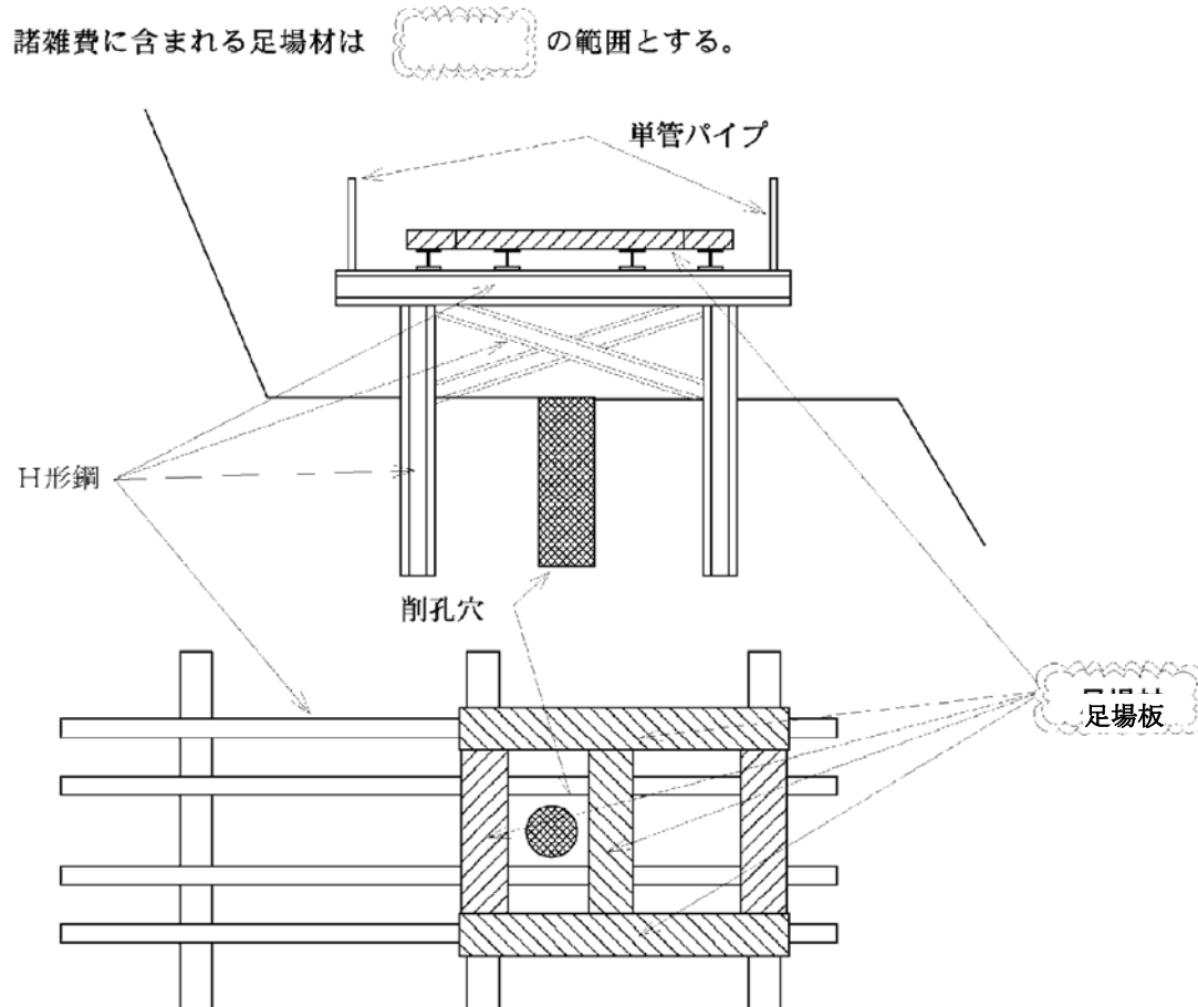
図 9-1 足場概念図
