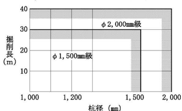
図 3-2 掘削機別選定
