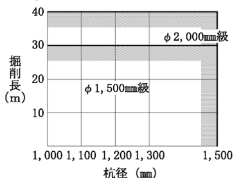
図 3-1 掘削機別選定
