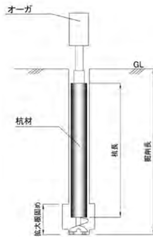
図 1-1 施工図（グラウト注入）
