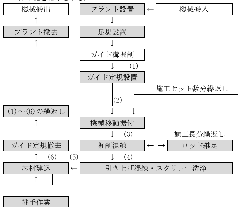
図 2-1 施工フロー
