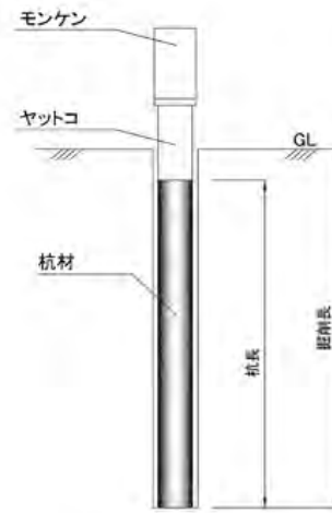
図 1-2 施工図（打撃）
