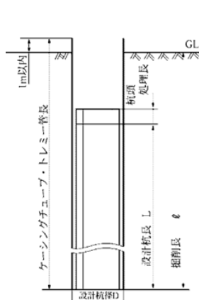
図 5-1 施工図（揺動式）
