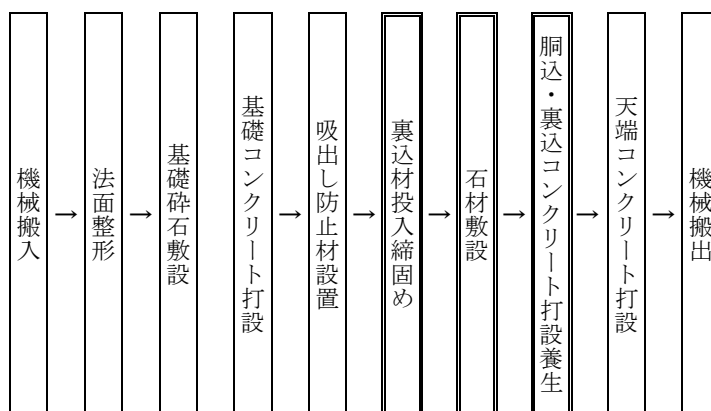
図 2-1 施工フロー
