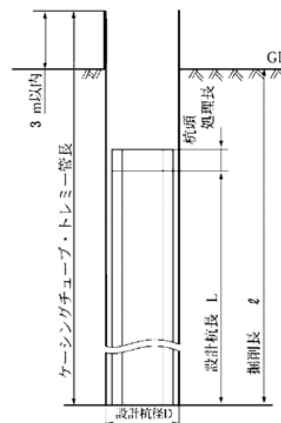
図 5-2 施工図（全回転式）
