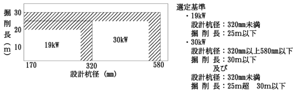
図3-2 大口径ボーリングマシンの選定
