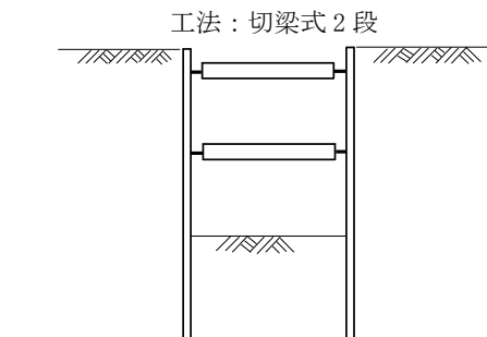
断面図
