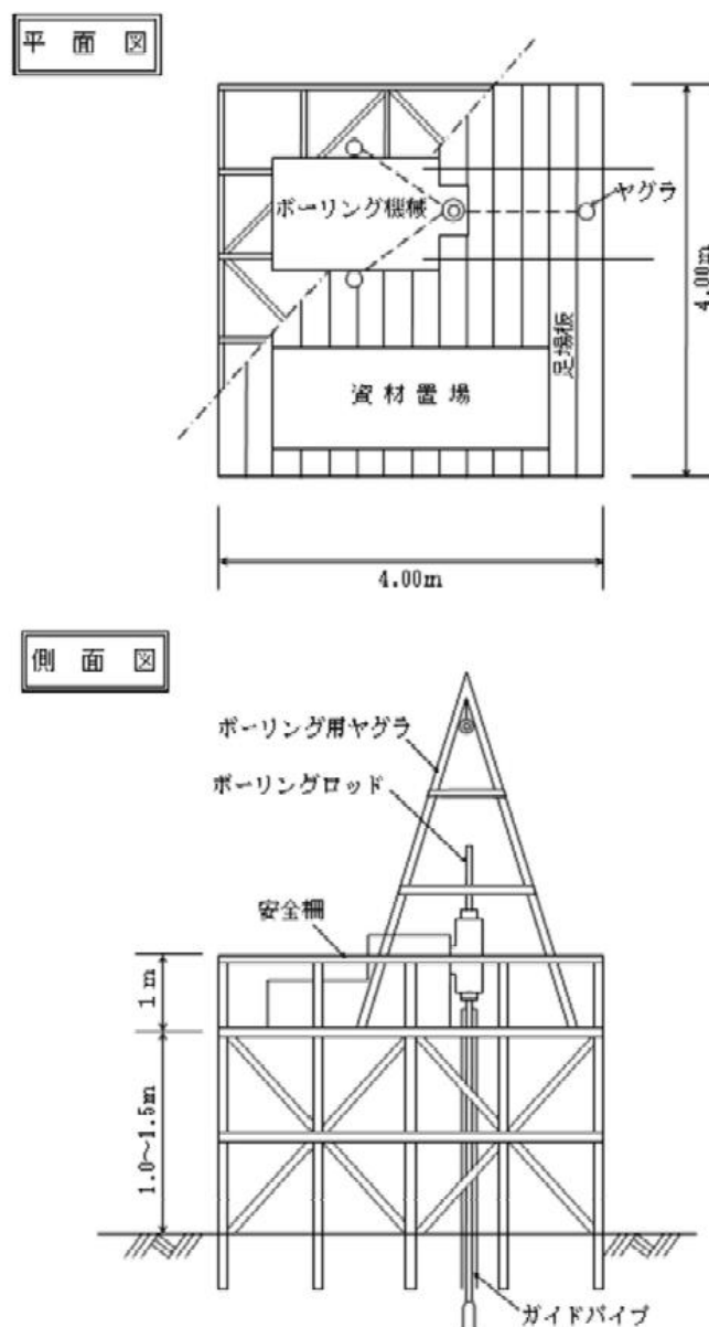
図 2-3-1 平坦地足場概念図
