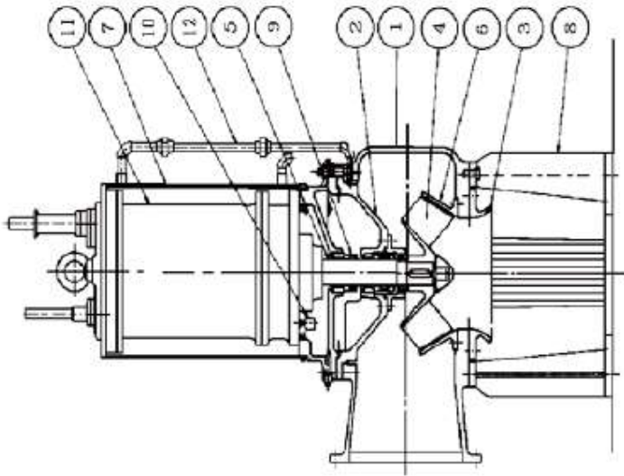
水中ポンプ(固定式)
