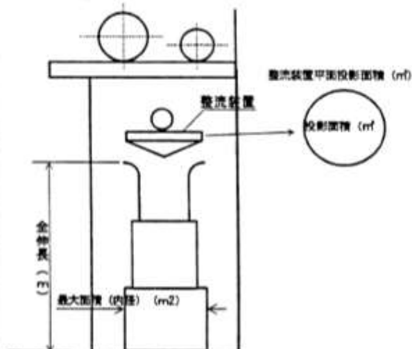
図-8 円形多段ゲート
