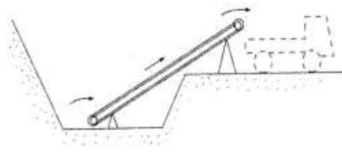
図 3. 2 傾斜据付
