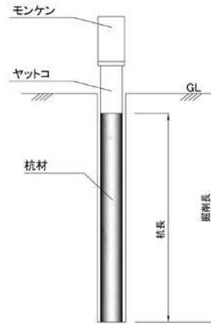
図 1-2 施工図（打撃）
