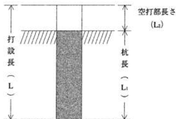
図 3-1 施工図
