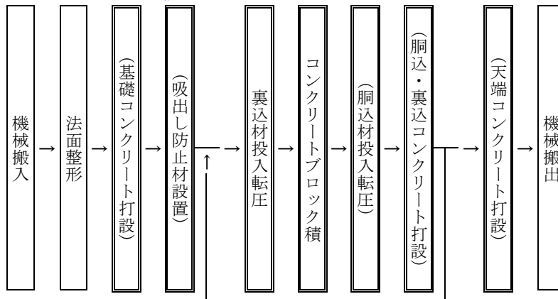
図 2-1 施工フロー（コンクリートブロック積工）
