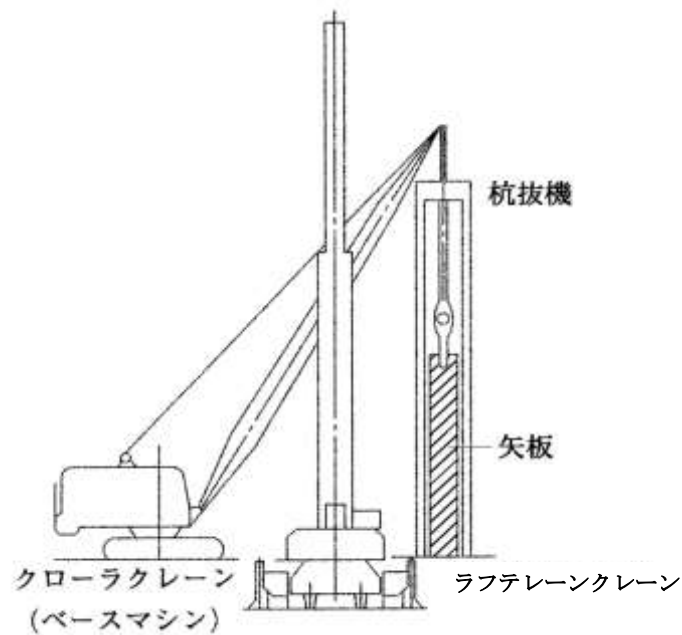
図 2-1 施工図
