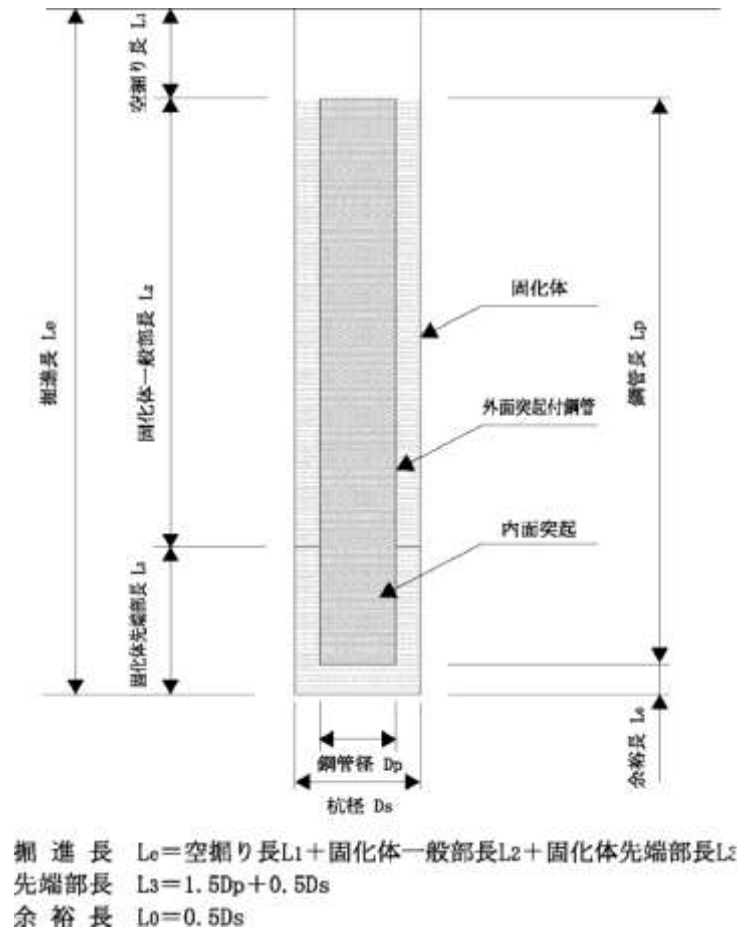
図 2.1 鋼管ソイルセメント杭のモデル図
