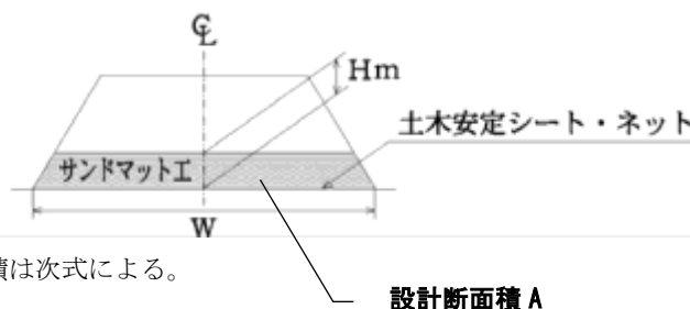
図 2-1 施工図
