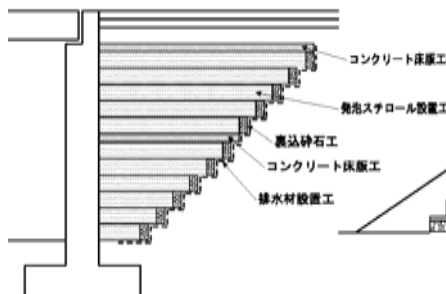
〔参考図3 (橋台裏込)〕
