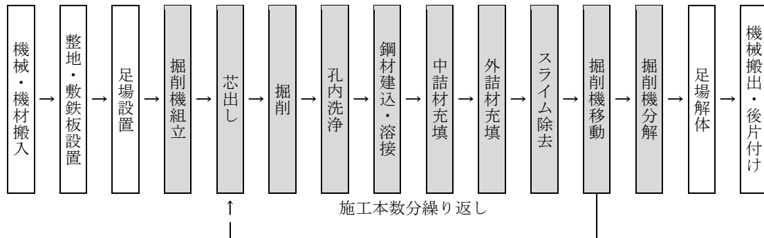
図 2-1 施工フロー
