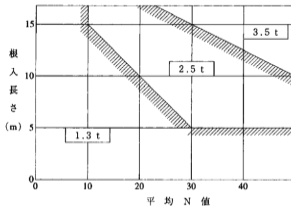
図 2.1 ディーゼルハンマ規格選定図
