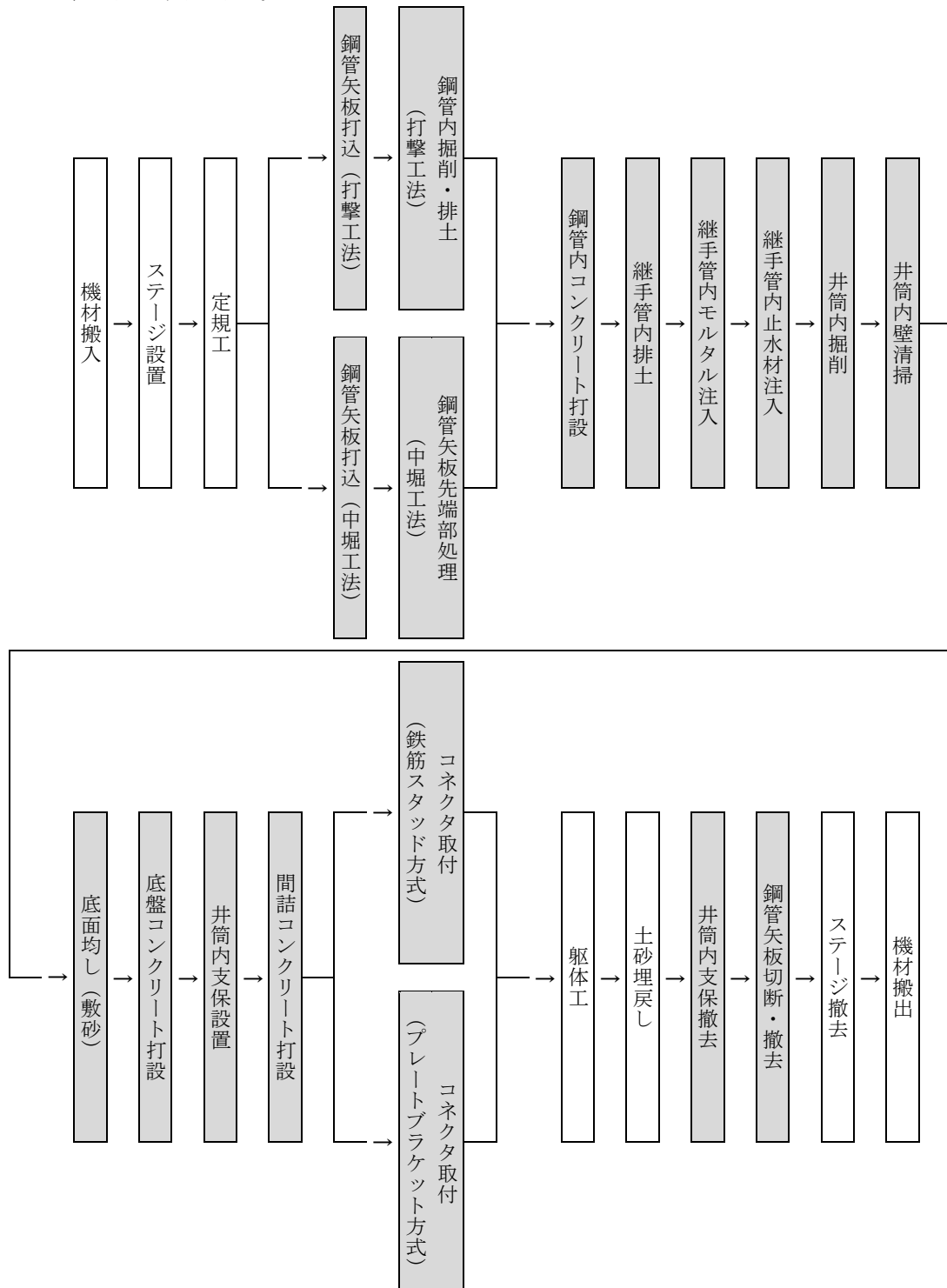
図 2.1 施工フロー
