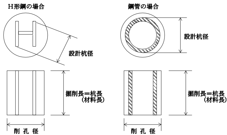
図 1-1 施工図
