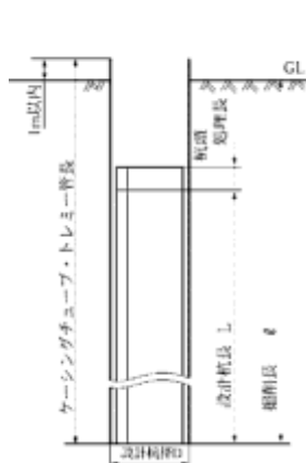
図 5-1 施工図（揺動式）
