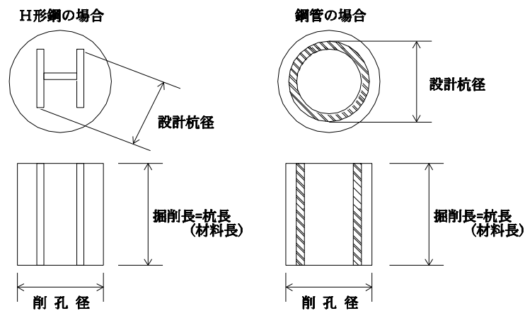
図 1-1 施工図
