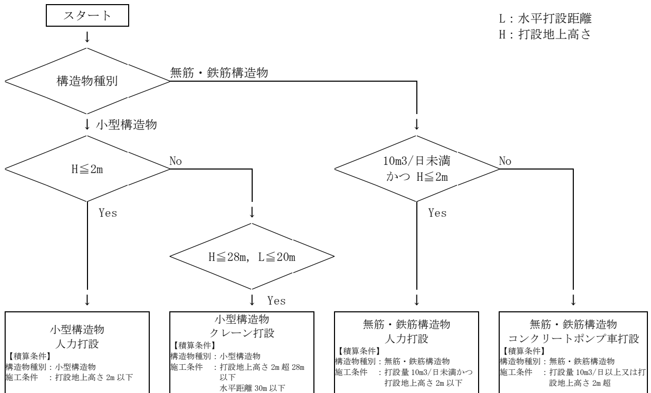
図 2.1 コンクリート打設工法の実定
