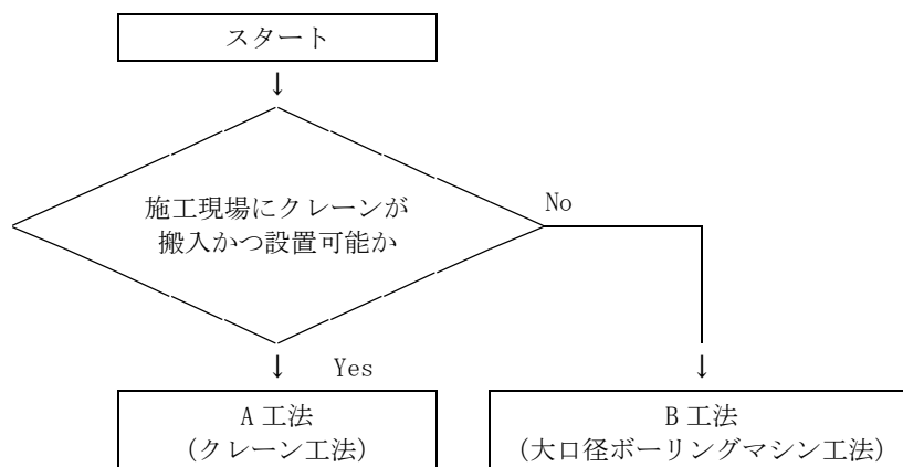
図 2-2 工法の選定
