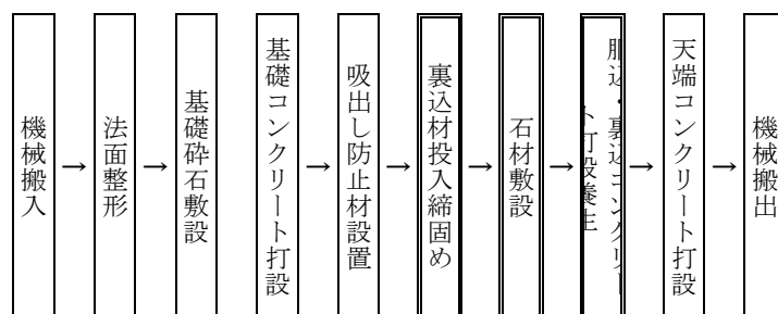
図 2-1 施工フロー
