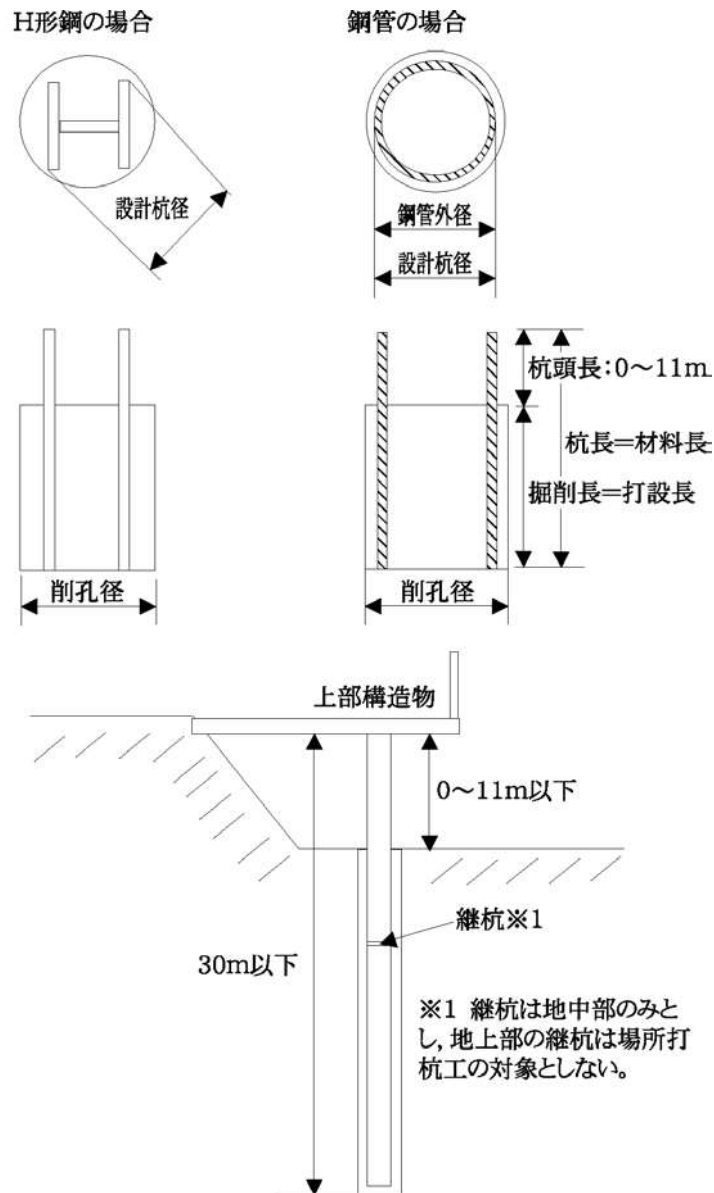
図 1-1 施工図
