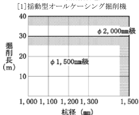
図 3-1 掘削機別選定
