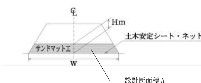
図 2-1 施工図
