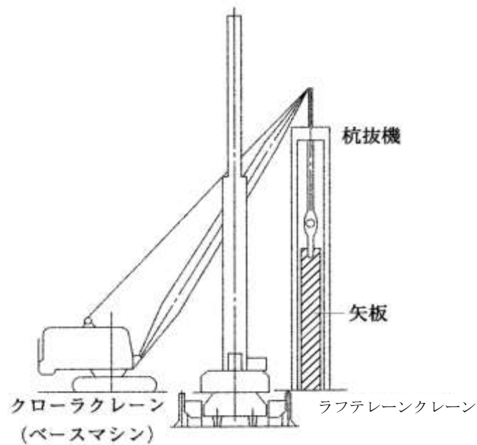
図 2-1 施工図
