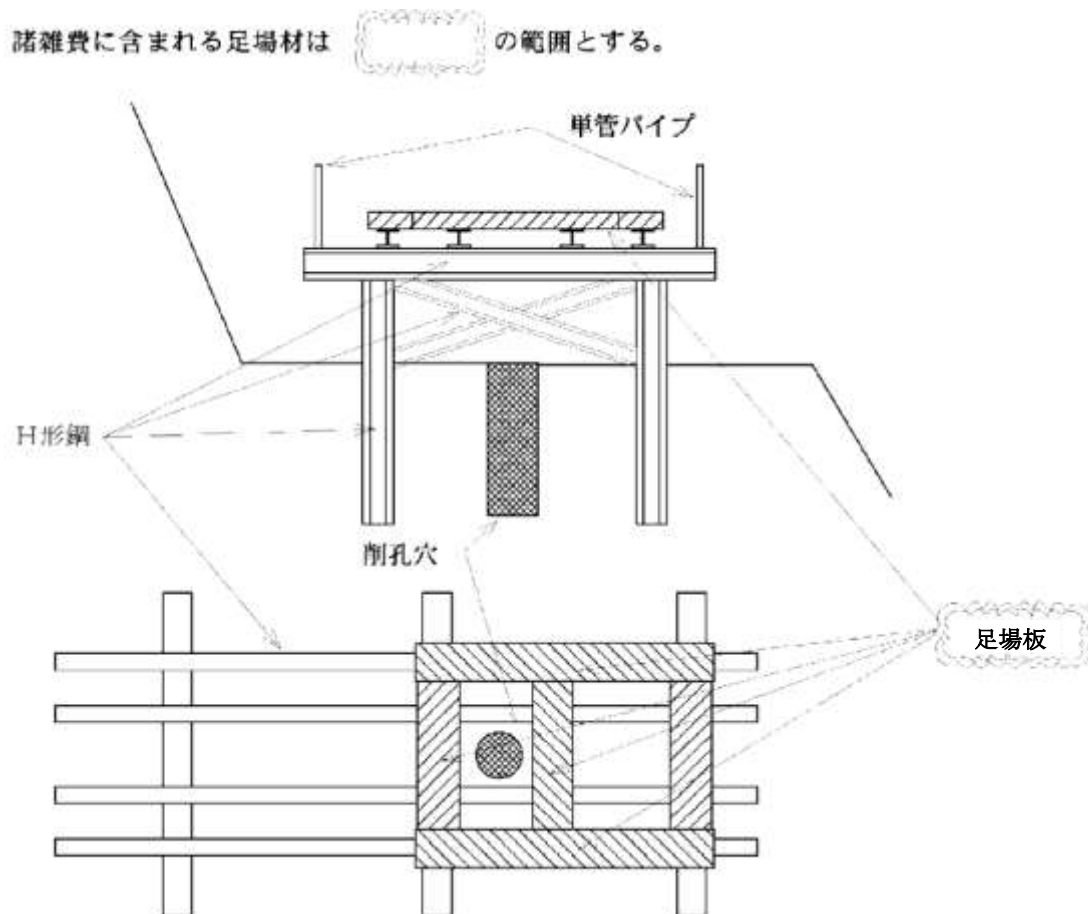
図 9-1 足場概念図
