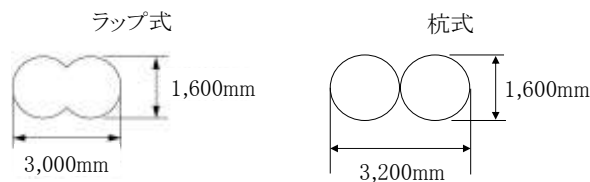
図 5-3 改良断面図
