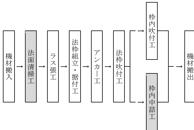
図 2-1 施工フロー
