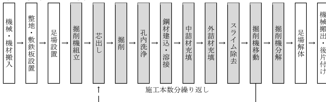
図 2-1 施工フロー
