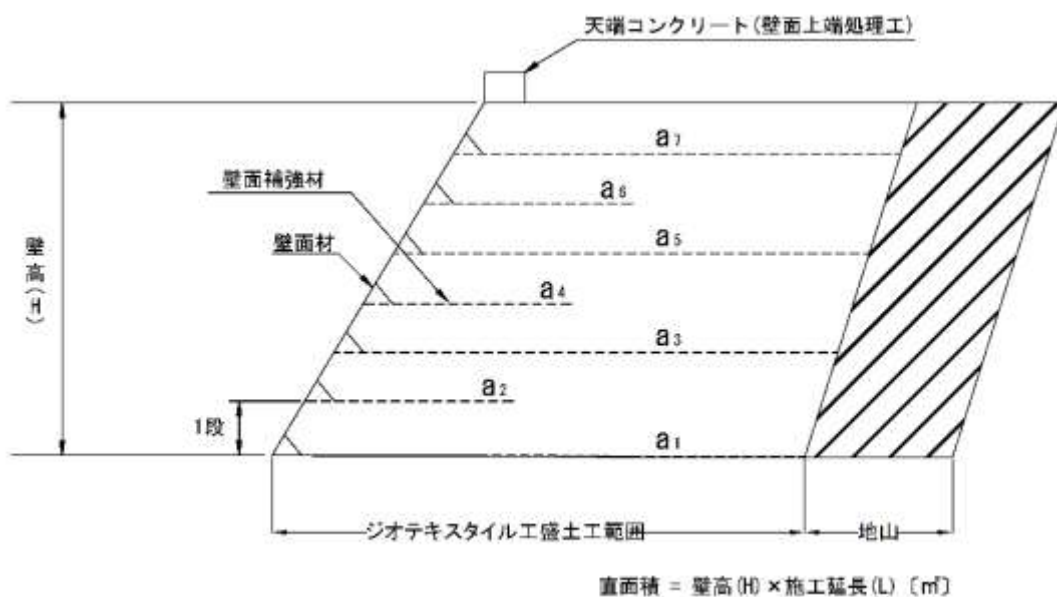
[参考図] ジオテキスタイル工標準断面図
