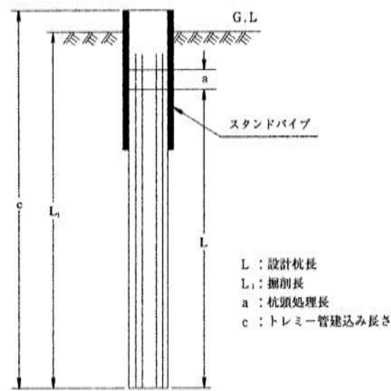
図 4-1 施工図
