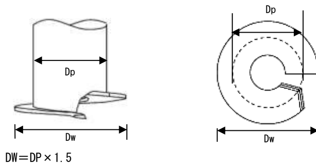
図 1-1 施工図
