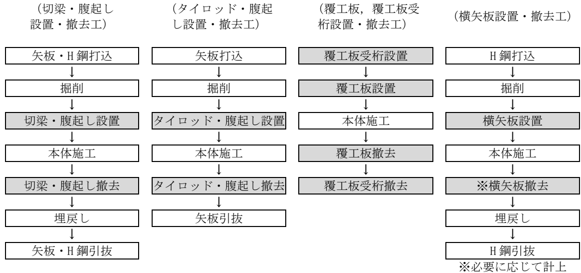
図 2-1 施工フロー
