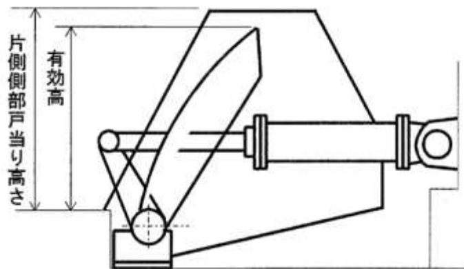
図-3 起伏ゲート
