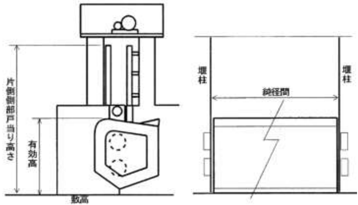
図-2 シェル構造ローラゲート
