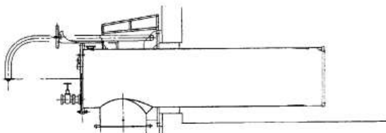
②コラムパイプ (右図) (付属品) ・吊り金具 ・ケープル押え ・0.5t手動チェーンブロック ・梯子 ・ケープル支持台 ・ケープルホルダ閉止蓋 ・コラムハッチ (締付ボルト含む) ・コラムハッチ引上装置 ・空気抜弁及びパイプ
