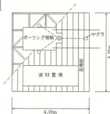
平面図
