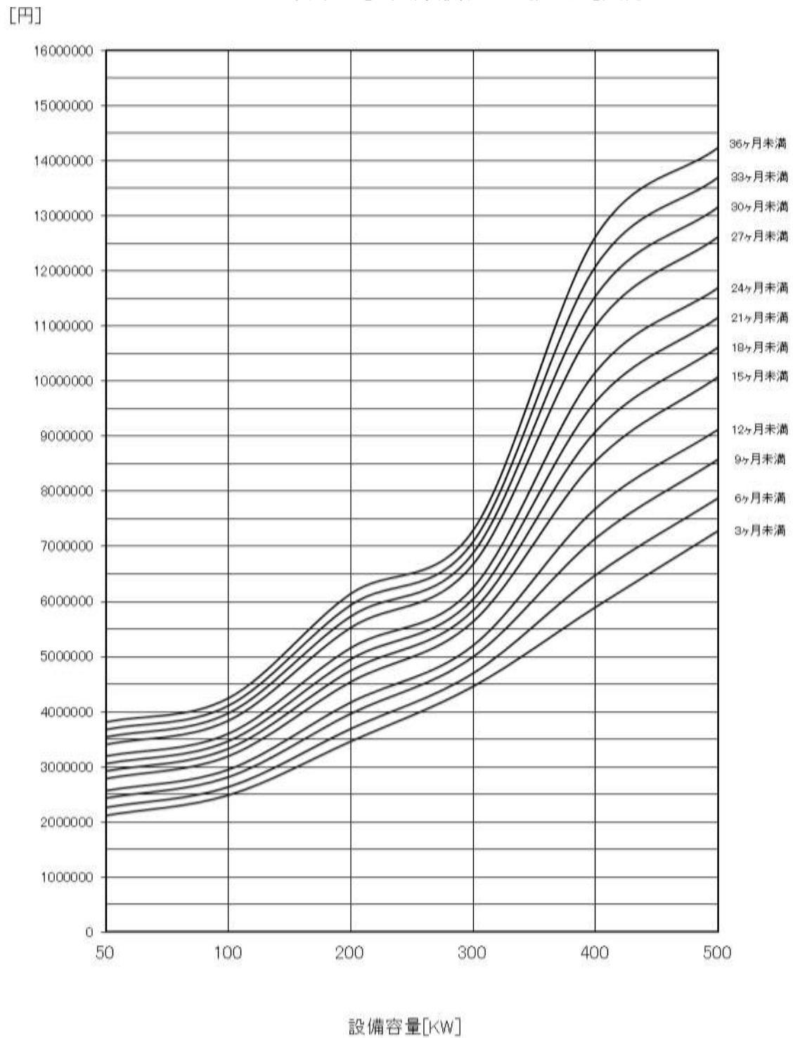
グラフ-(2) 土木工事仮設用電力設備費積算グラフ[高圧受電設備]
