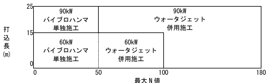
図 3-1 電動式バイブロハンマ機種の選定範囲
