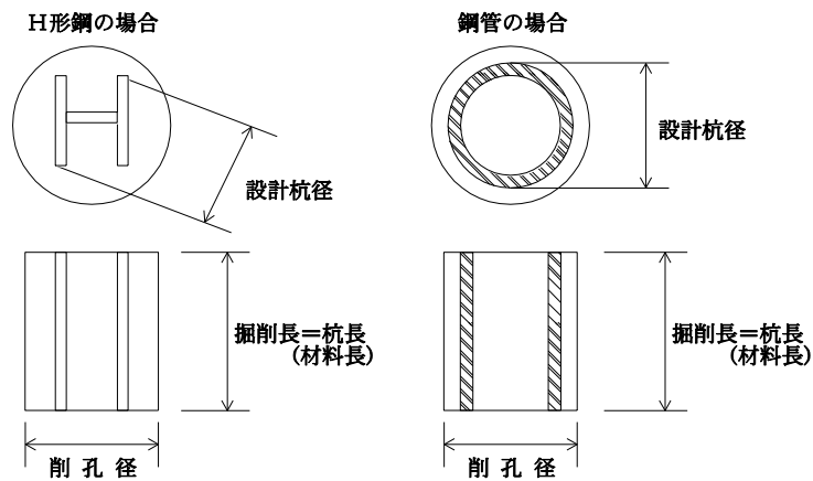
図 1-1 施工図
