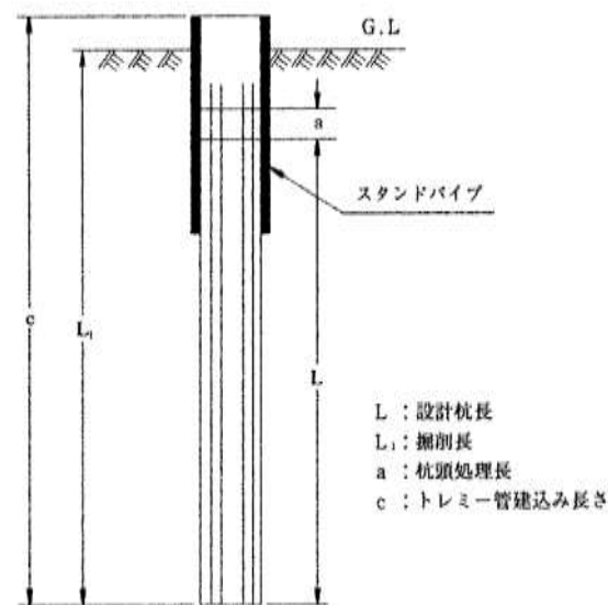
図 4-1 施工図
