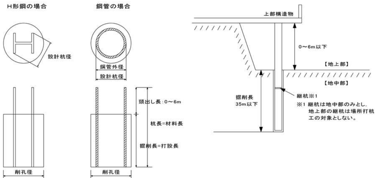
図 1-1 施工図
