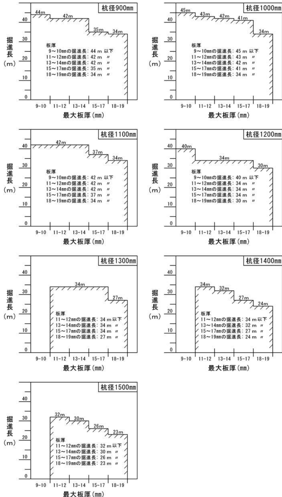
図 1-1 適用掘進長
