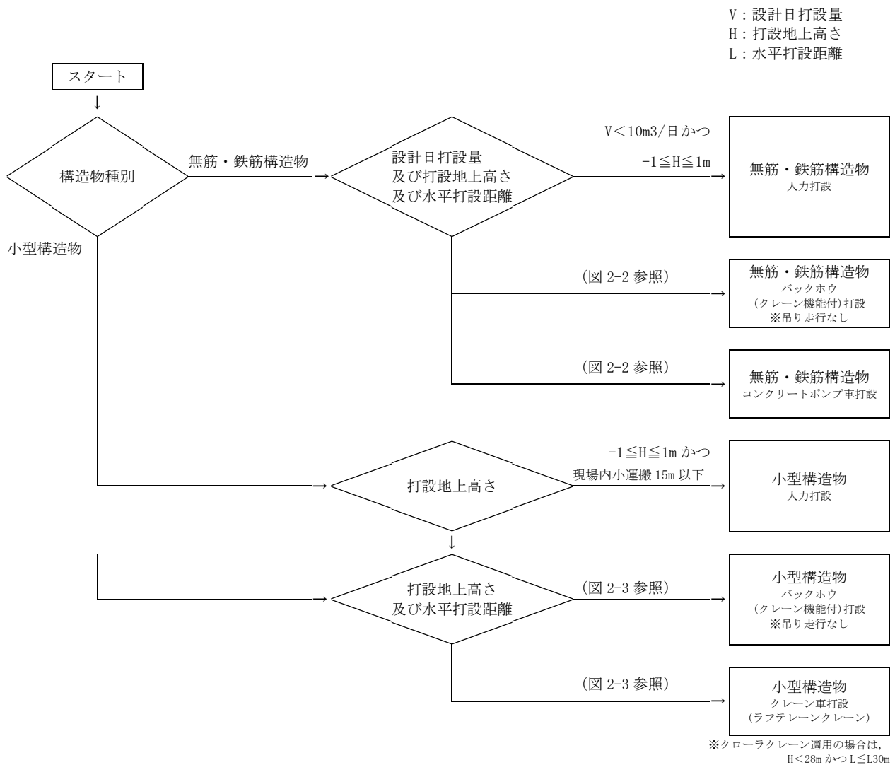
図 2-1 コンクリート打設工法の選定
