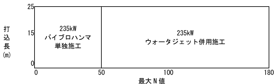
図 3-2 油圧式バイブロハンマ機種の選定範囲
