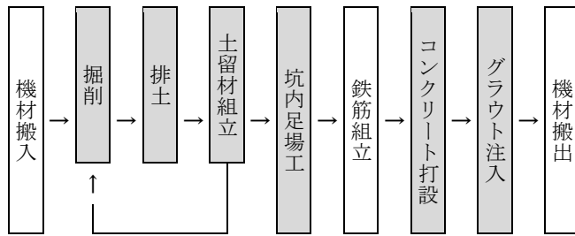
図 2-1 施工フロー
