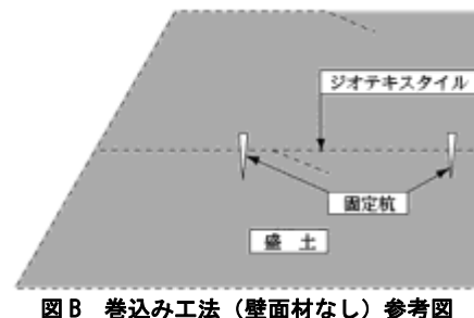
図 B 巻込み工法（壁面材なし）参考図
