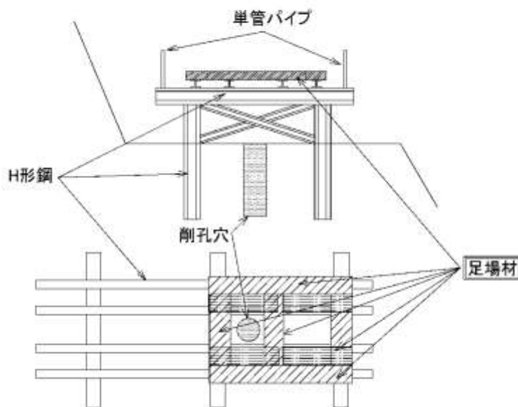
図 9-1 足場概念図
