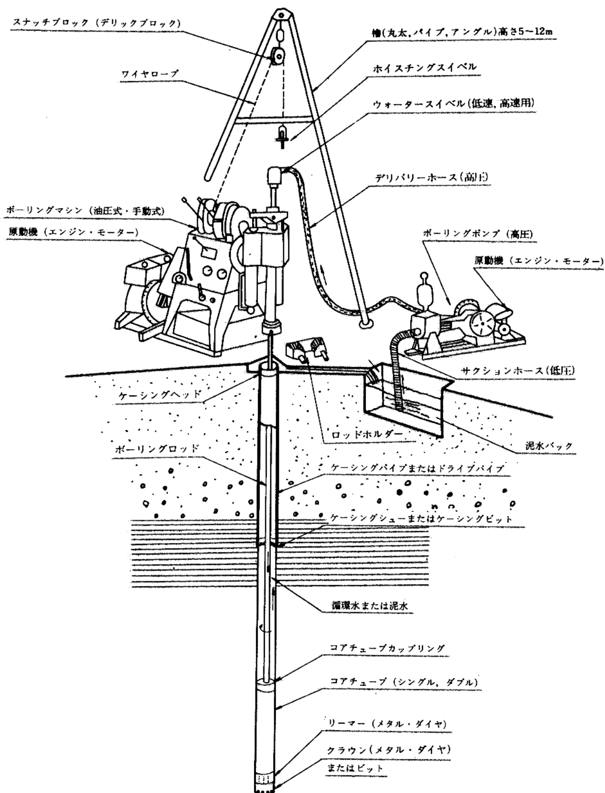
図 2-1-1 設備概念図
