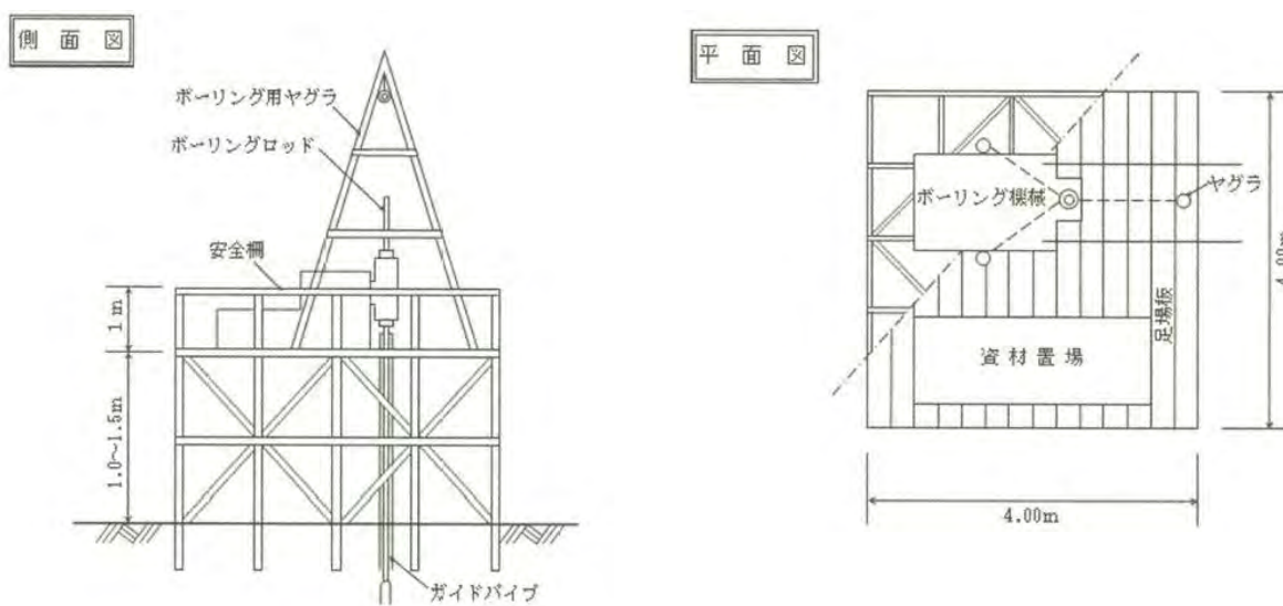
（嵩上げ足場）
