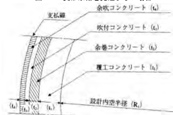
図 3.11 変形余裕を見込まない場合
