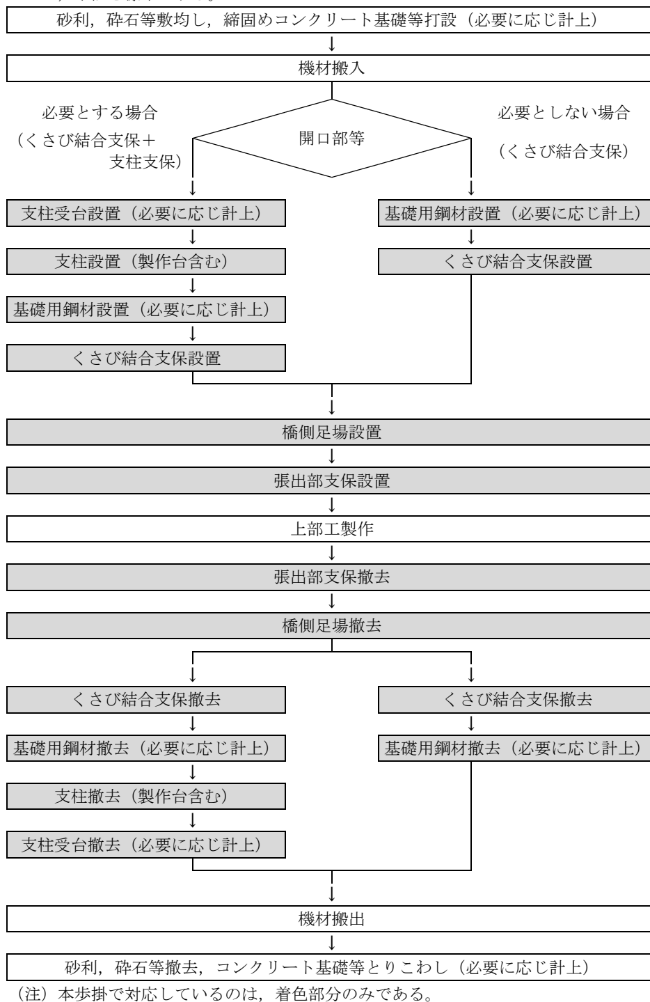
図 2-1 施工フロー
