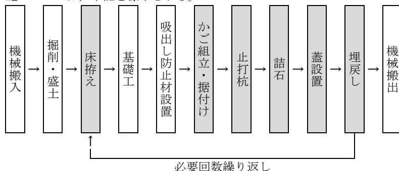
図 2-1 施工フロー
