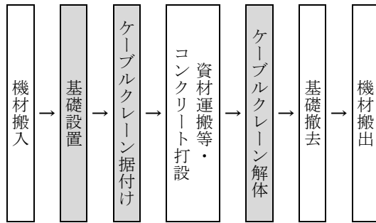
図 1-1 施工フロー
