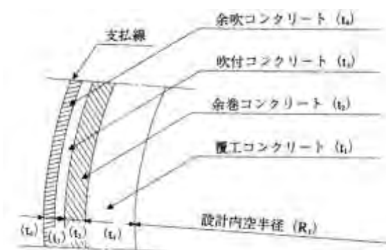
図 3.1 変形余裕を見込まない場合
