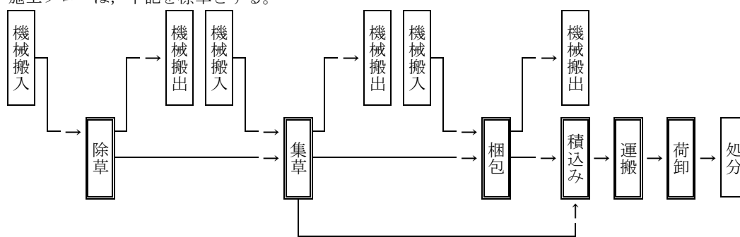
図 2-1 施工フロー
