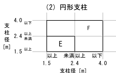
図 1.2 円形支柱の適用範囲
