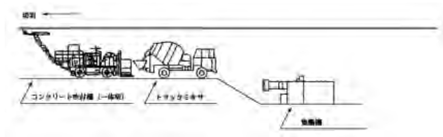
図 4.1 吹付コンクリート施工機械配置例 (参考図)
