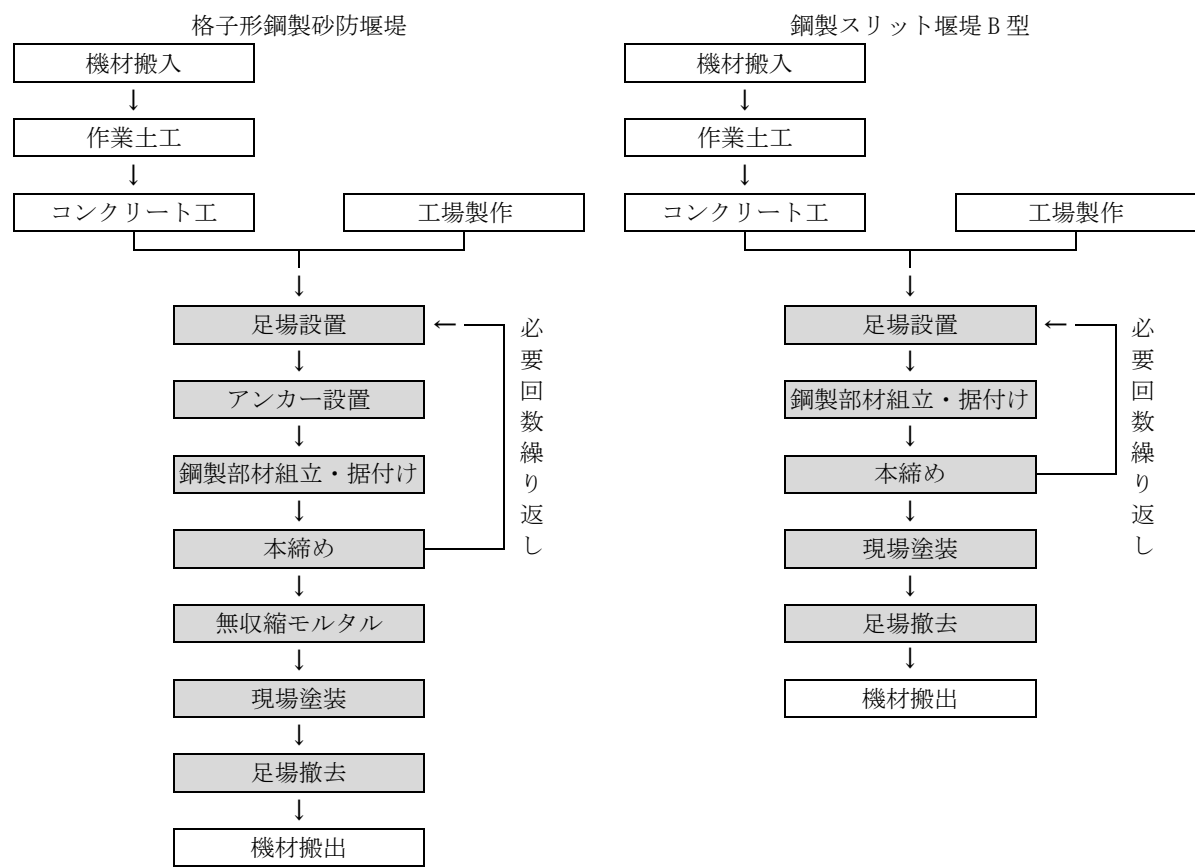
図 2-1 施工フロー
