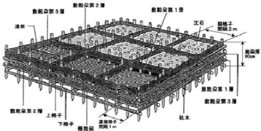
図 3-1 参考図（粗朶沈床概念）
