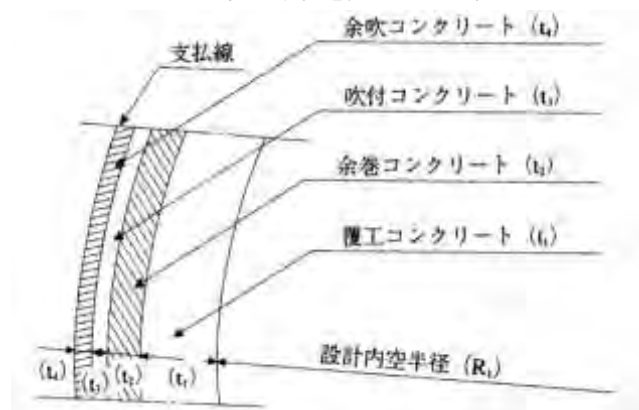
図 3.6 変形余裕を見込まない場合
