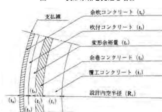
図 3.12 変形余裕を見込む場合
