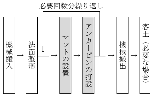
図 2-1 施工フロー
