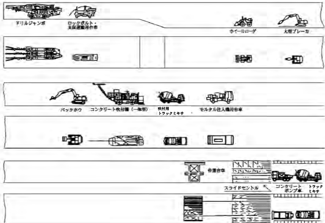
図 3.10 上半先進ベンチカッタ工法（上下半交互併進工法）
