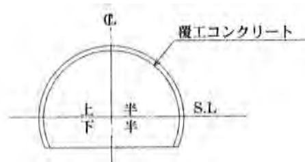
図 1.1 加背割図
