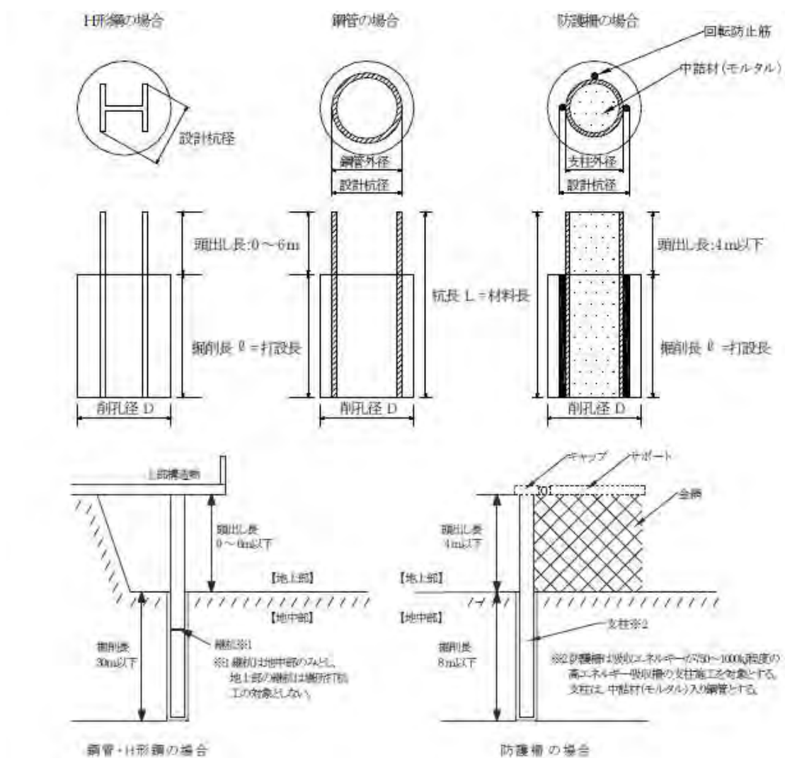
図 1-1 施工図
