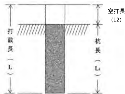
図 3-1 施工図
