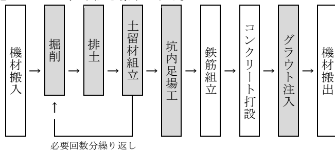
図 2-1 施工フロー
