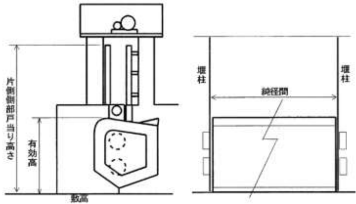
図-2 シエル構造ローラゲート
