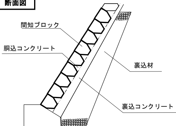
断面図
