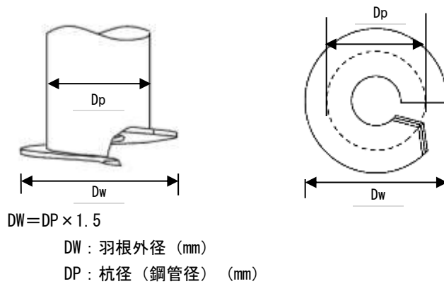
図 1-2 羽根の概要図（開口タイプ）
