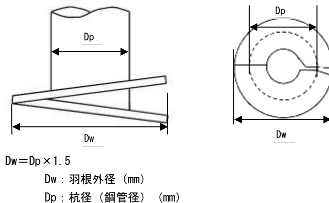
図 1-3 羽根の概要図（開端タイプ）
