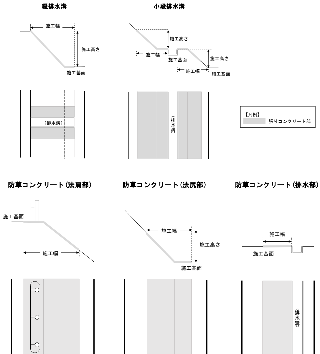
図 1-1 張りコンクリートの例
