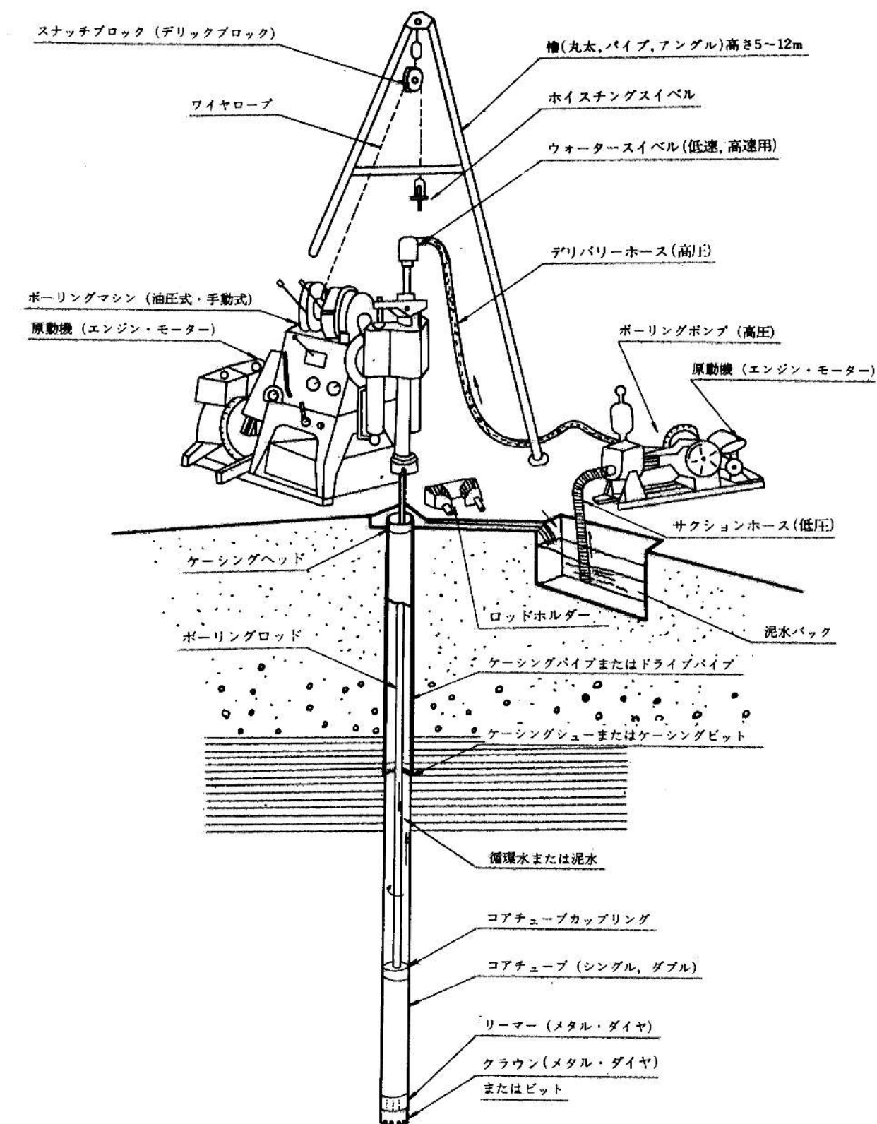
図 2-1-1 設備概念図
