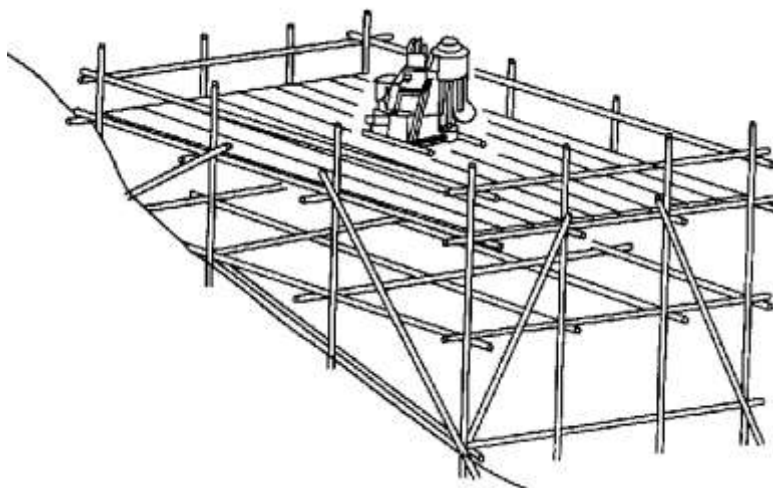
図 2-3-3 傾斜地足場概念図
