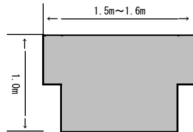
参考図 各工種の標準壁面形状
