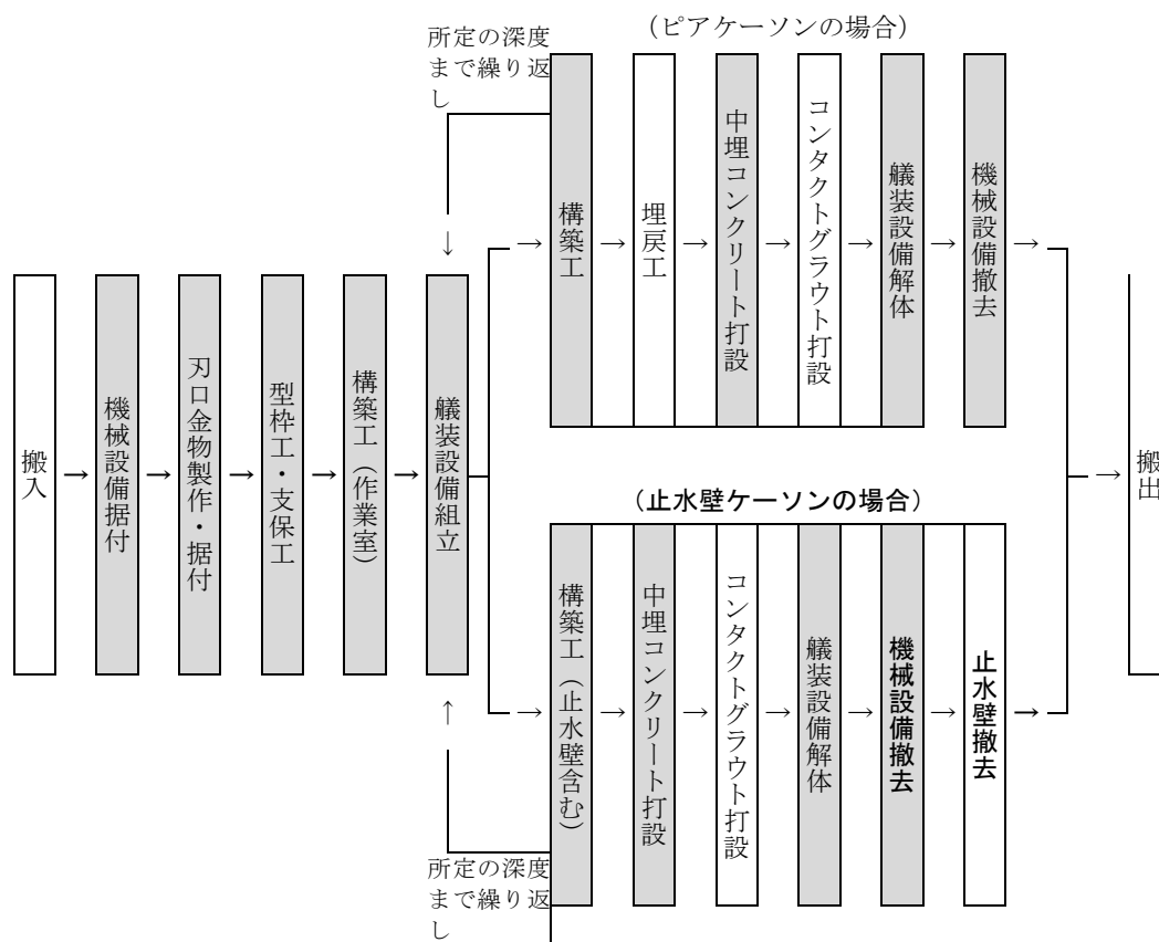
図 2-1 施工フロー
