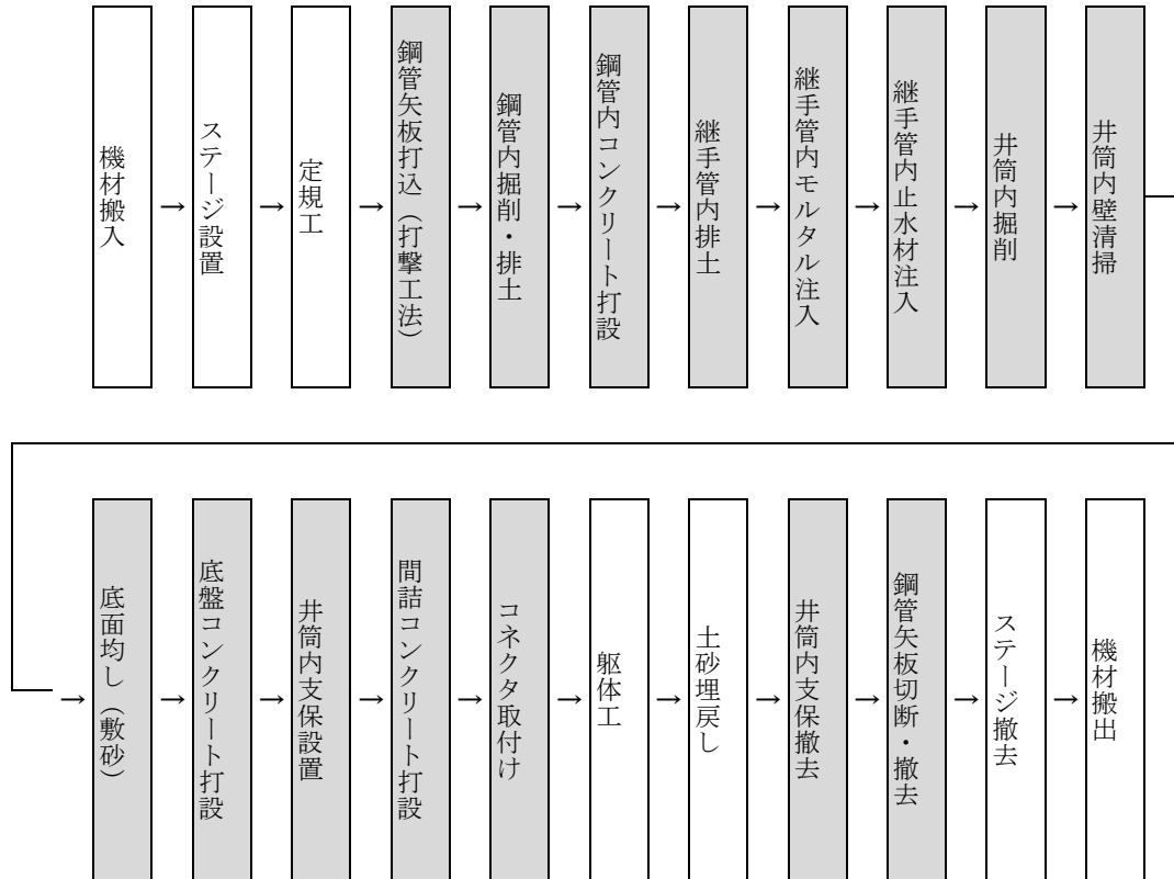
図 2-1 施工フロー
