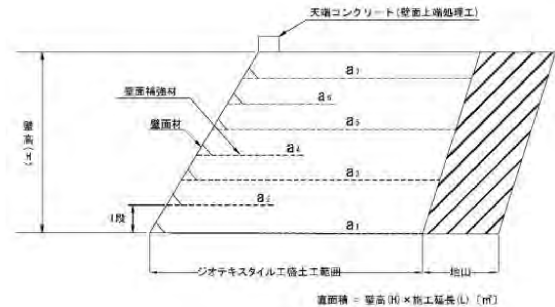
[参考図] ジオテキスタイル工標準断面図
