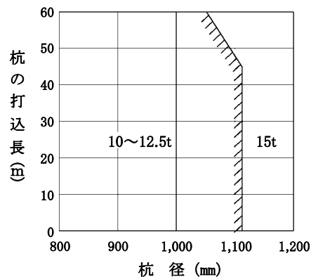
図 3-1 油圧パイルハンマの選定
