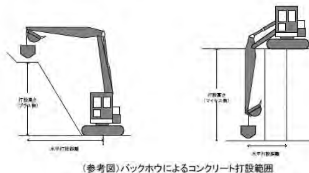
図 3-3 コンクリート打設工法の選定（小型構造物）
