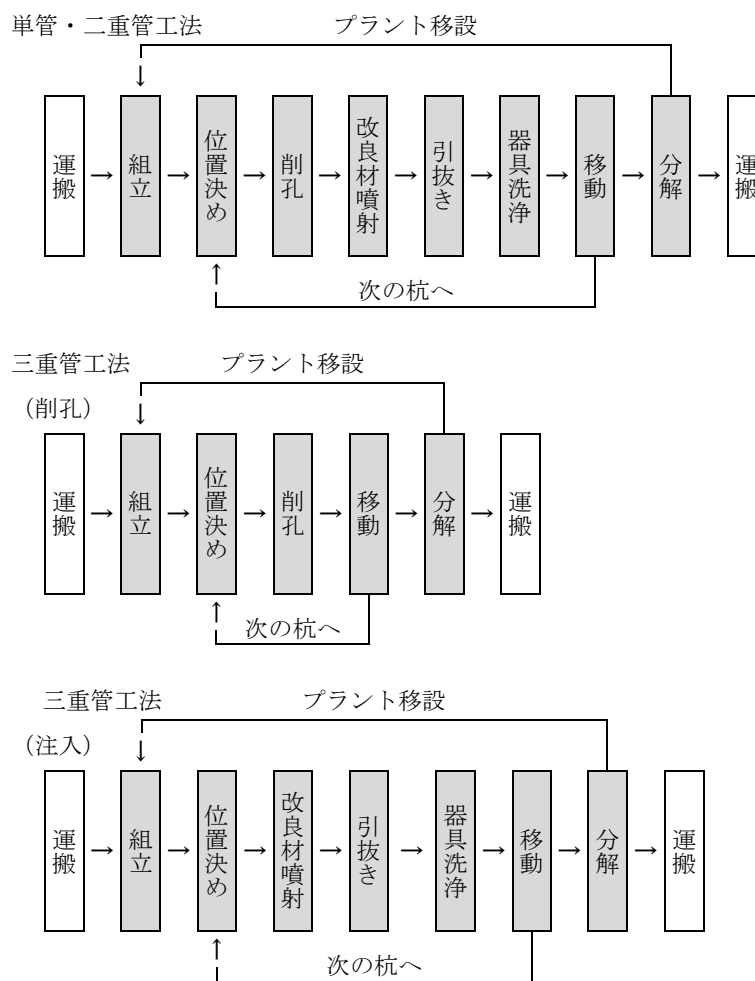
図2.1 施工フロー図
