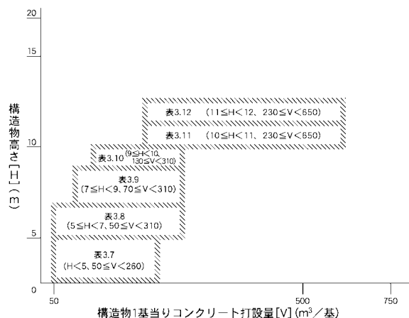
図 3-2 壁式橋脚步掛表適用範囲
