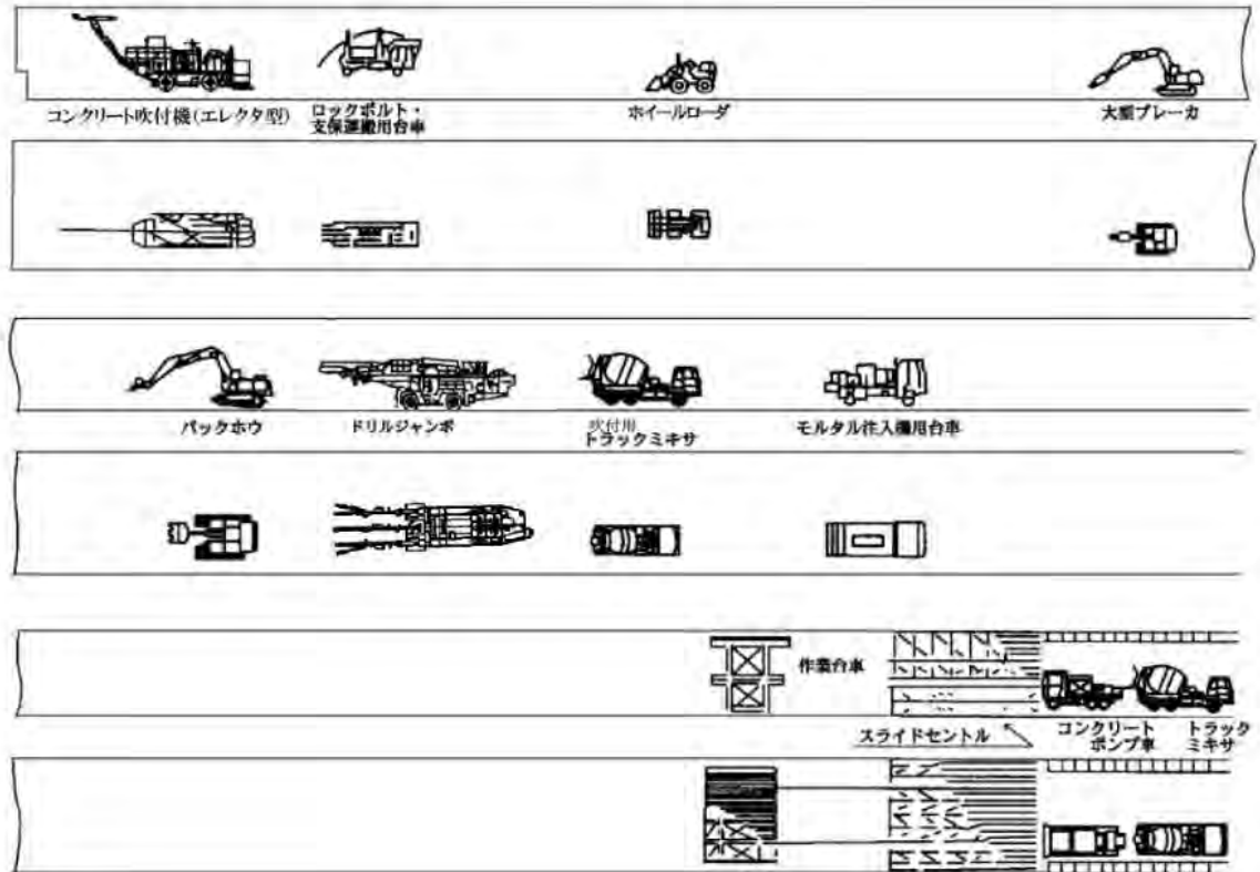
図 3.5 補助ベンチ付全断面工法
