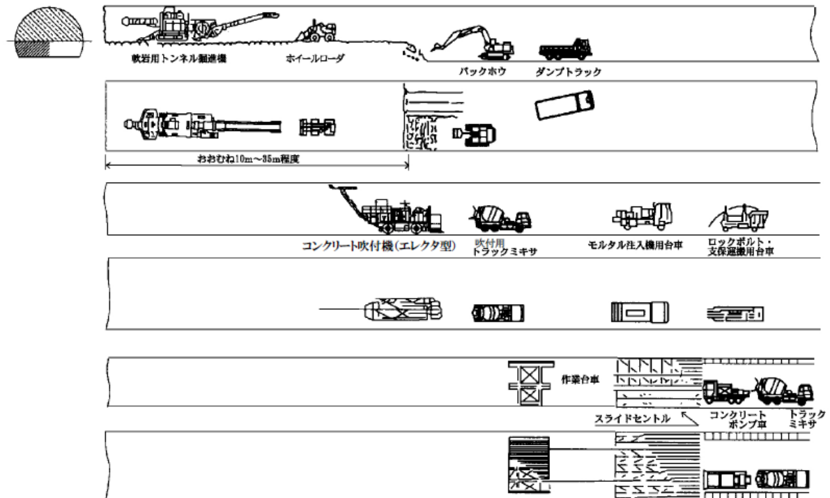
図 3.2 上半先進ベンチカット工法（上下半同時併進工法）
