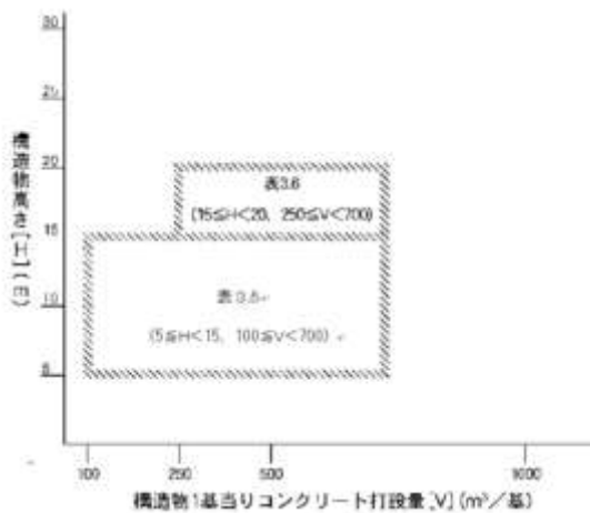
図 3-1 T 形橋脚步掛表適用範囲
