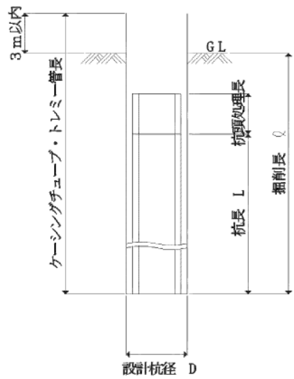
図 5-1 施工図
