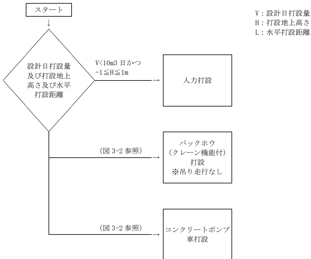
図 3-1 コンクリート打設工法の選定（1）
