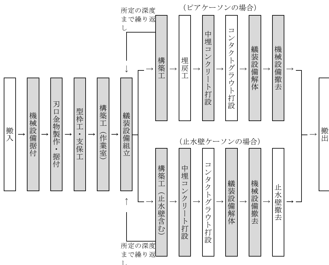
図 2-1 施工フロー
