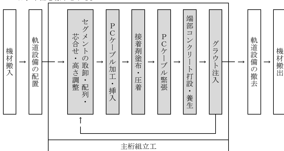
図 2-1 施工フロー
