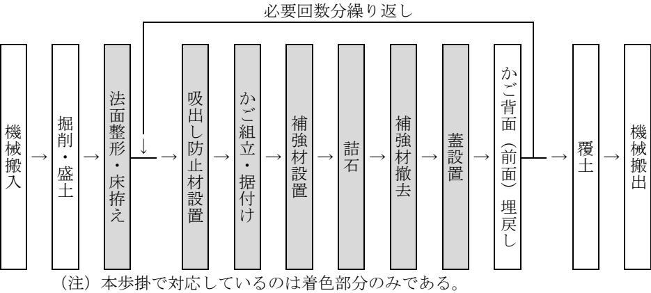
図 2-1 施工フロー
