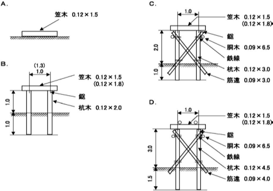
図 5-2 受枠の構造図
