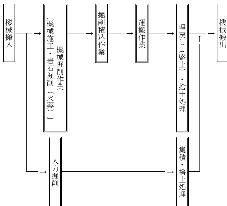
図 2-1 施工フロー
