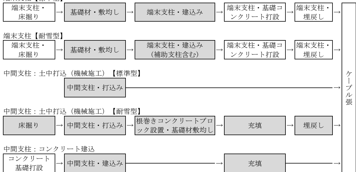
図 2-1 施工フロー
