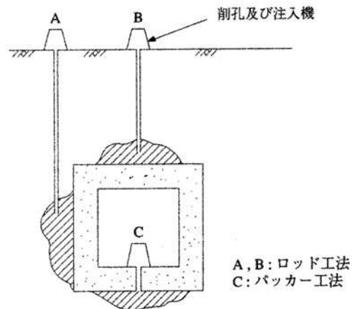
图 1-1 施工法
