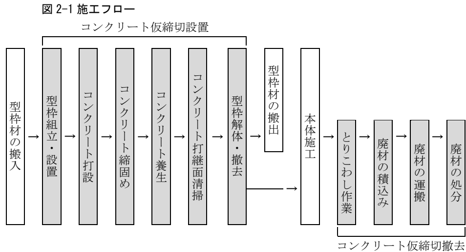
図 2-1 施工フロー
