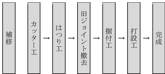
図 4-2 施工フロー（既製品ジョイント）
