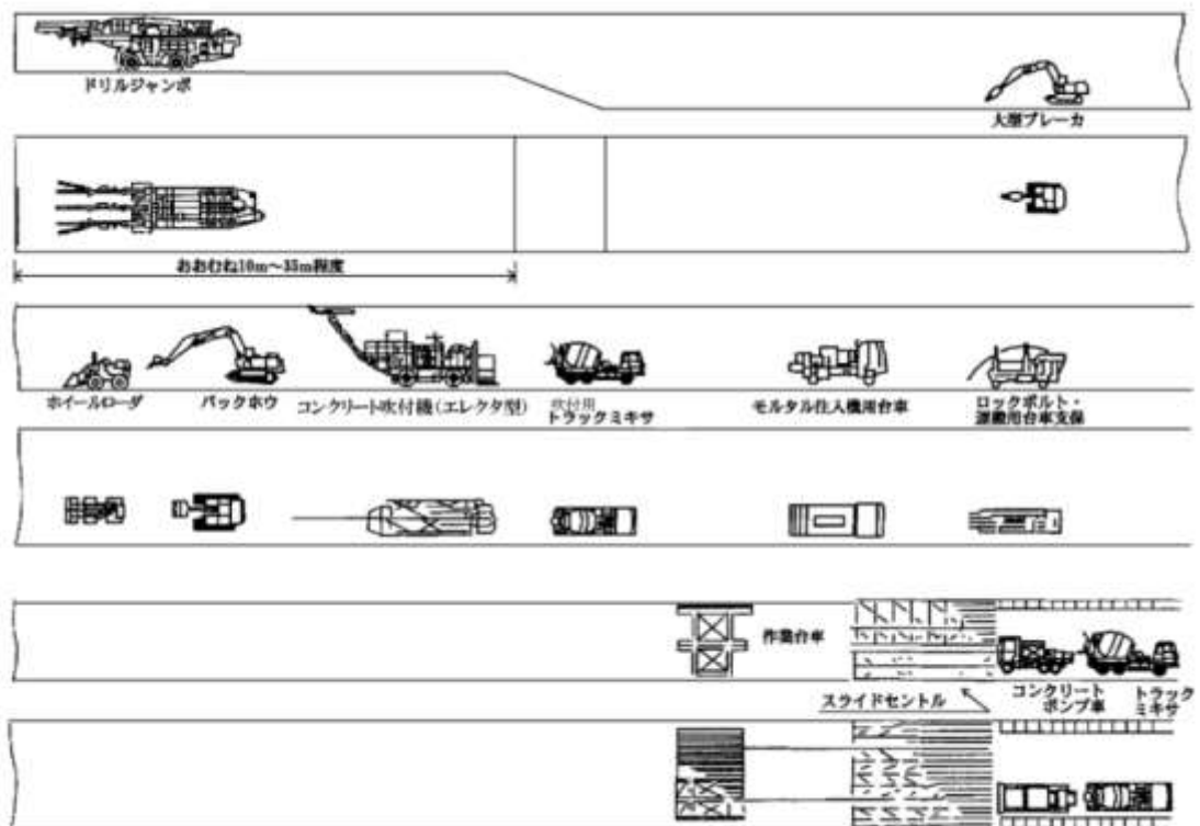
図 3.9 上半先進ベンチカット工法（上下半交互併進工法） 掘削機械配置例（4）（上半ロックボルト作業時）
