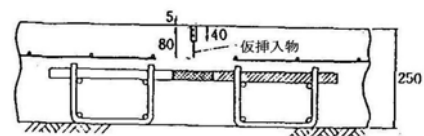
打込み目地で仮挿入物とカット切断による場合
