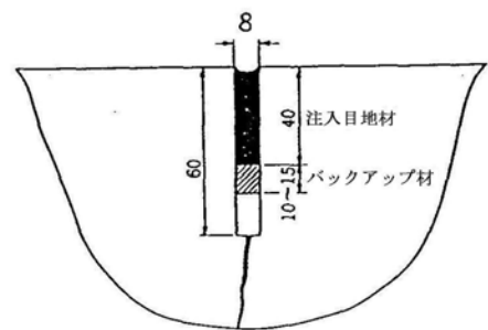
カット目地に用いるバックアップ材の例 (単位: mm)
