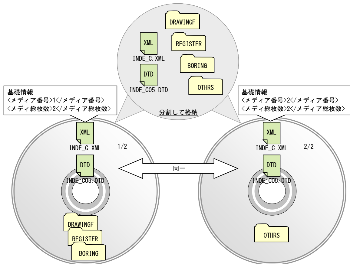
図 5-19 電子媒体が2枚になる場合の作成（例）
