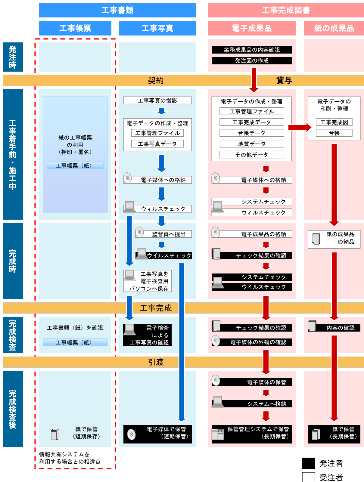
図 2-1 土木工事における電子納品・電子検査の流れ (紙の工事帳票を利用する場合)
