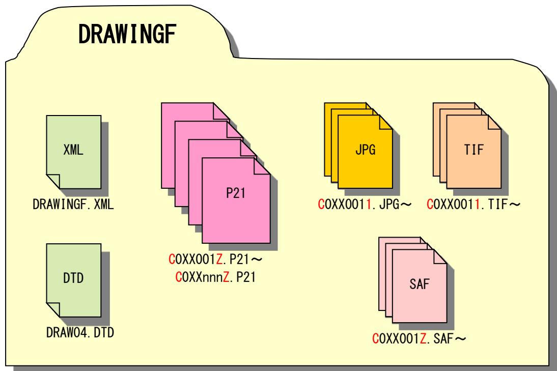
図 5-7 工事完成図フォルダ（DRAWINGF）の格納イメージ（SXF Ver. 3.0 の場合）
