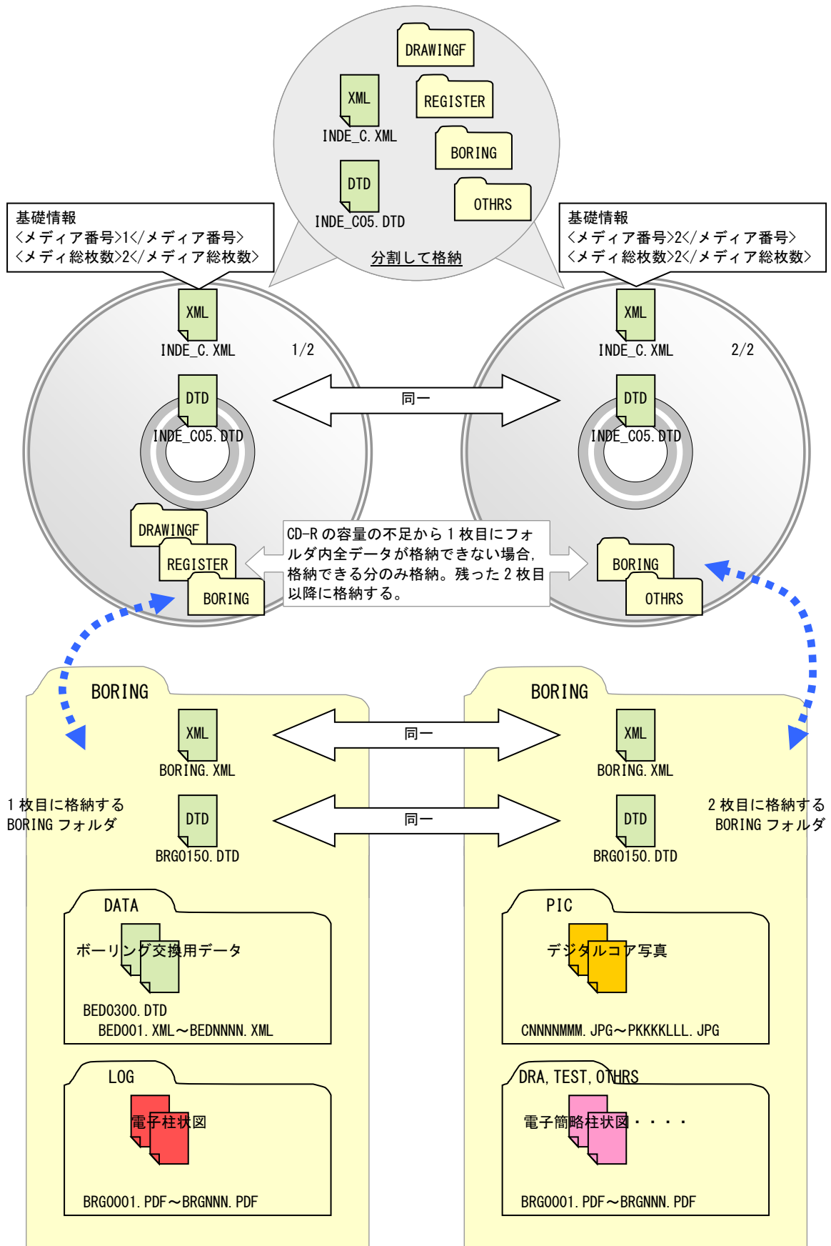
図 5-20 電子媒体が 2 枚になる場合の作成（例）【フォルダを分割する場合】
