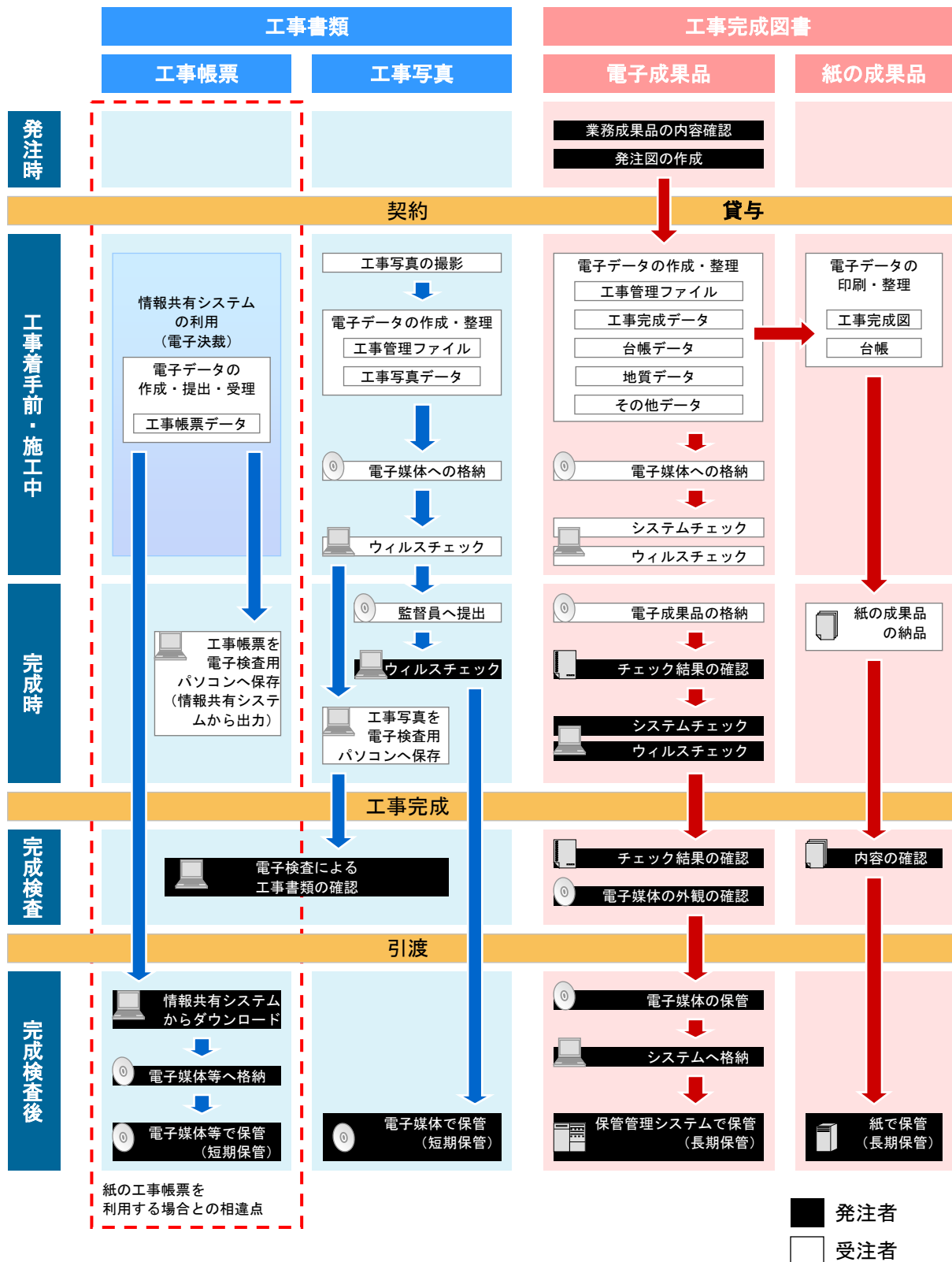
図 2-2 土木工事における電子納品・電子検査の流れ (情報共有システムを利用する場合)
