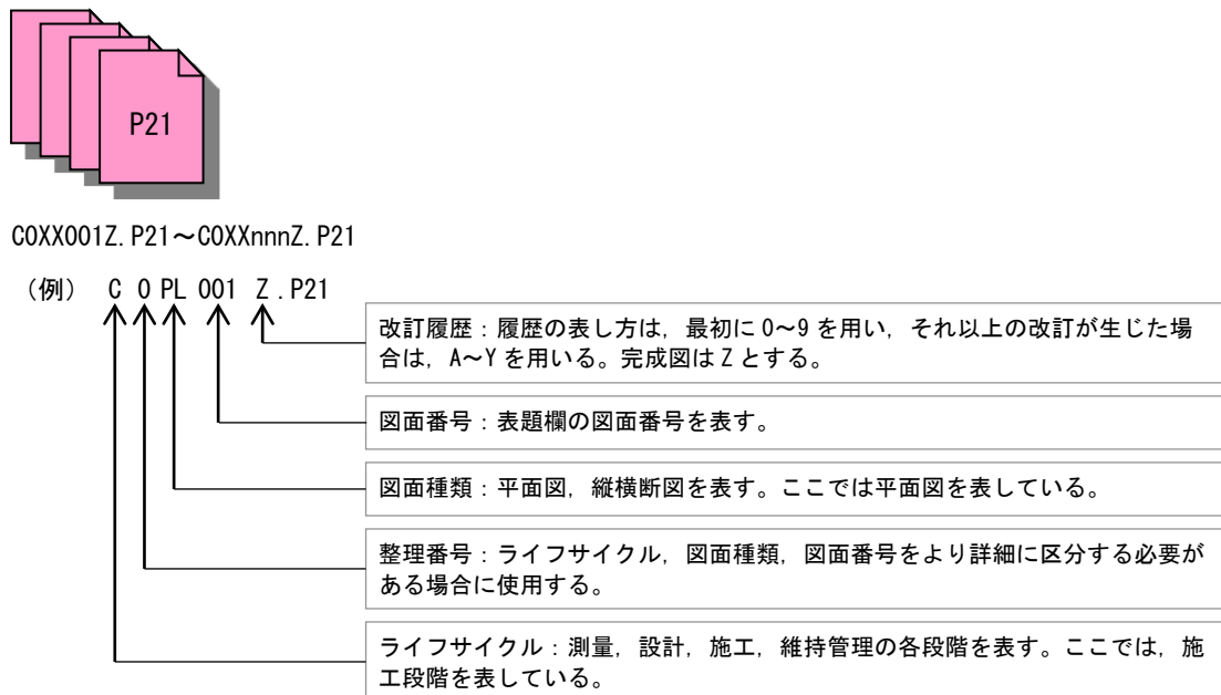
図 5-6 工事完成図ファイルの命名（例）
