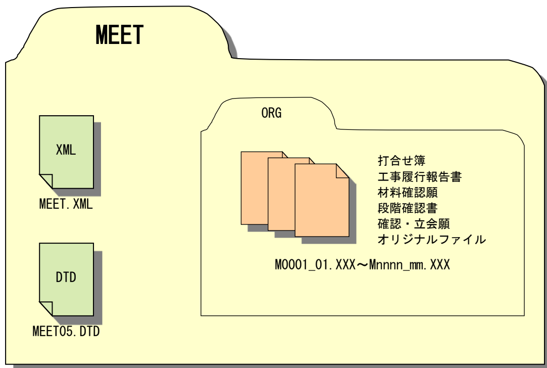
図 7-6 打合せ簿フォルダ（MEET）の格納イメージ
