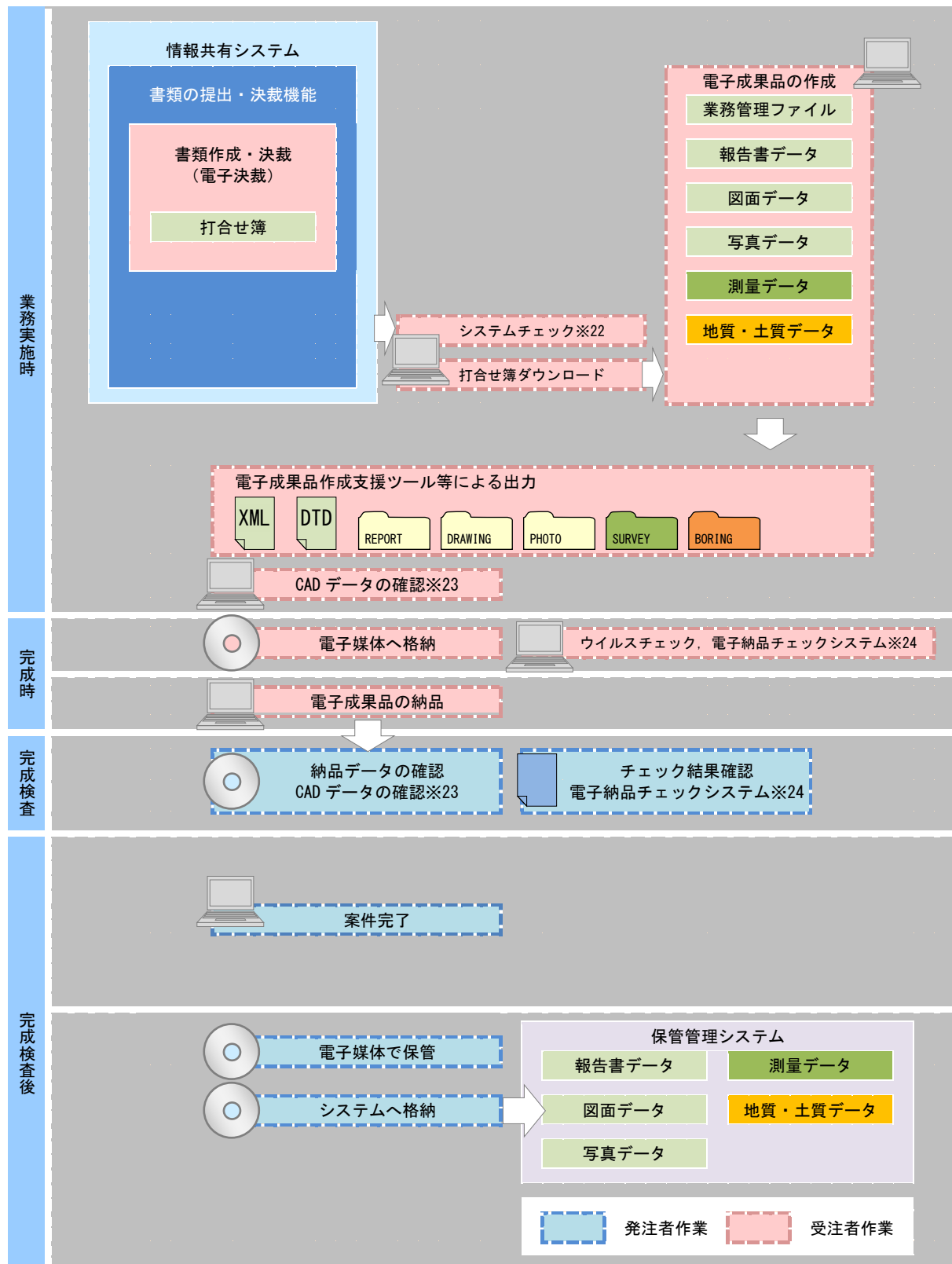
図 9-2 情報共有システムを利用した電子成果品の流れ
