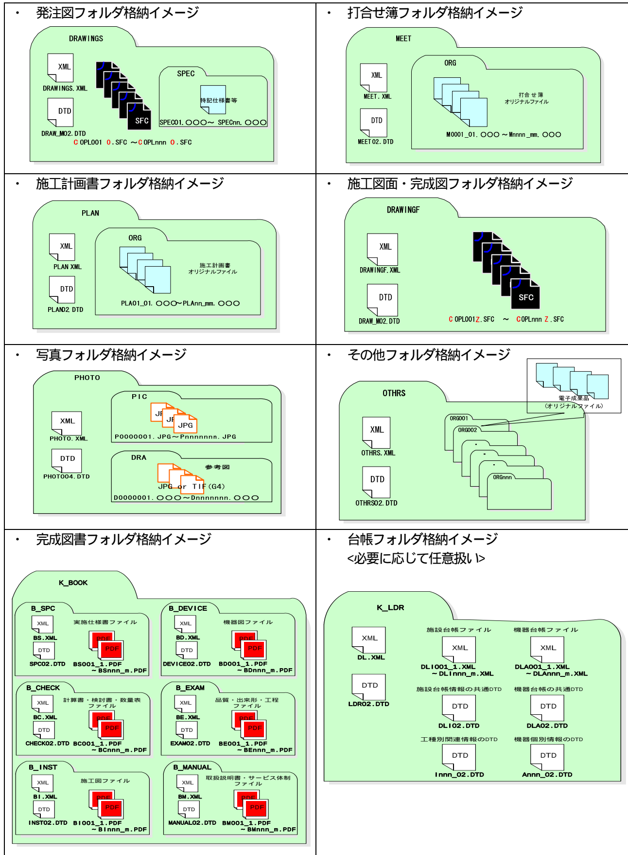
図 5.6 フォルダ構成(電子媒体 CD-R , DVD-R)及び各フォルダの格納・整理イメージ
