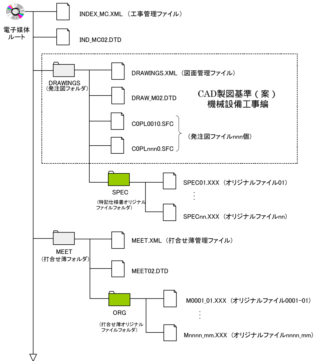
図 5.1 フォルダ構成(1/5)
