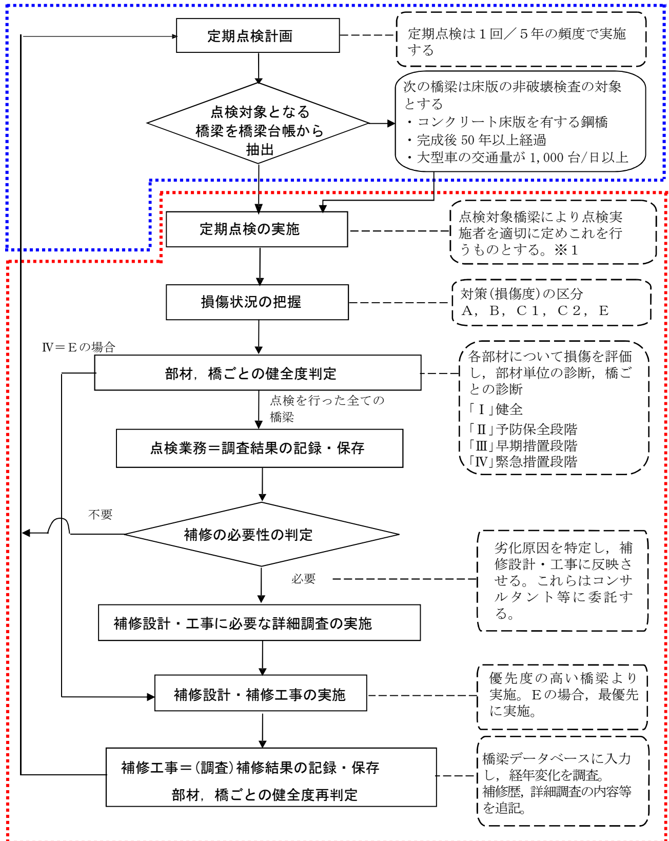
図2.1 橋梁定期点検実施フロー
