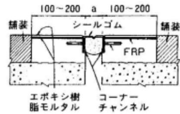
突き合わせ後付形式の例
