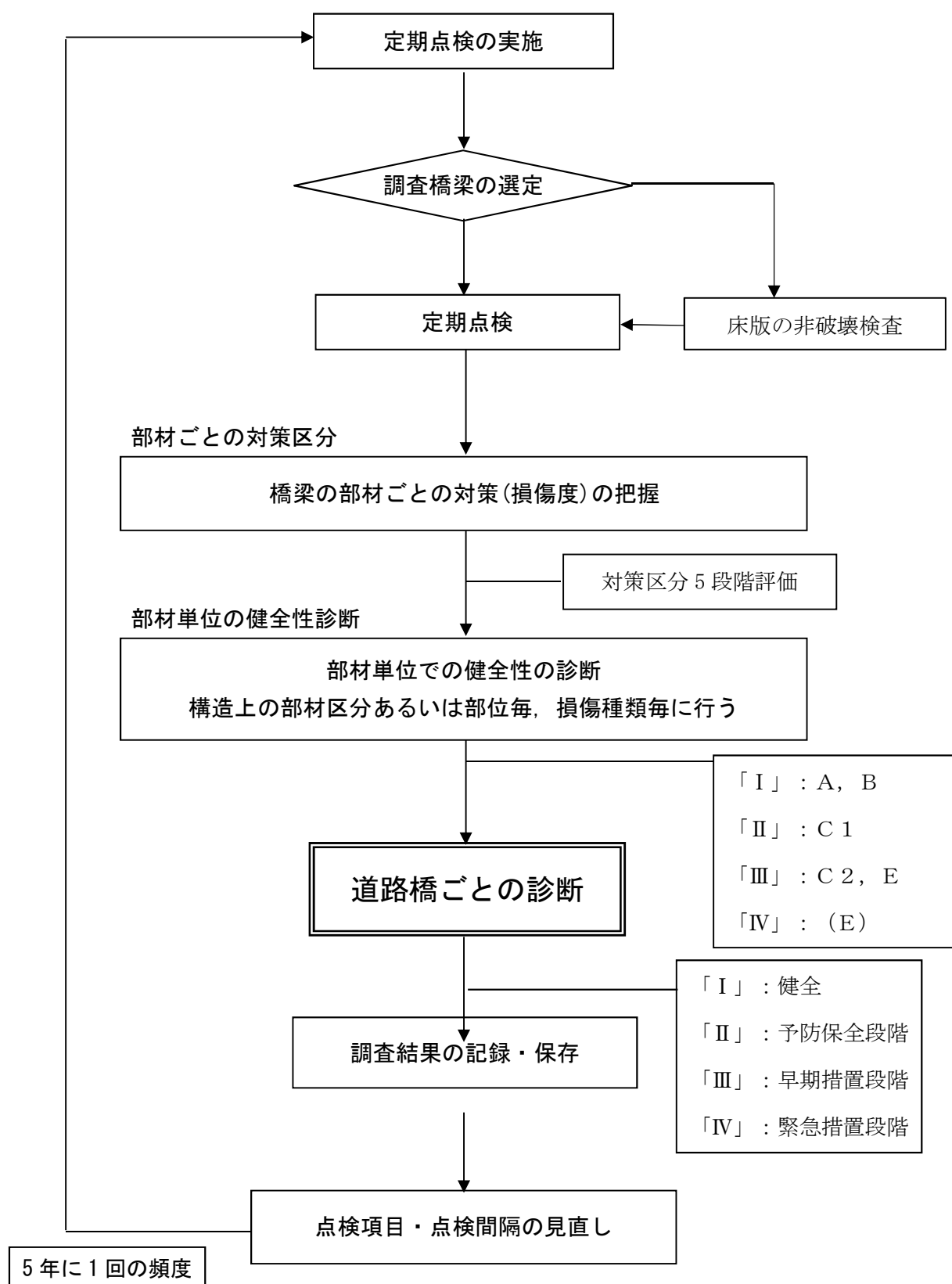
図3. 1 定期点検業務 判定フロー
