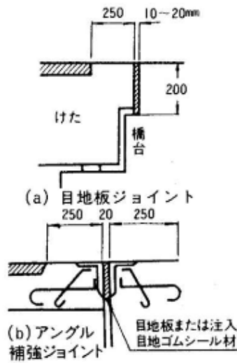
突き合わせ先付形式
