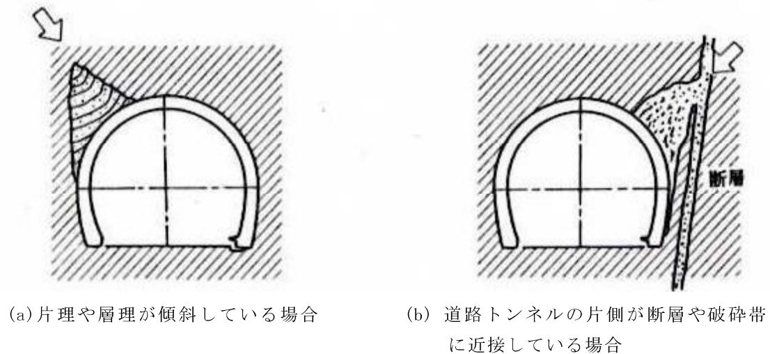
図 5 層状岩盤の周辺の偏土圧の模式図
