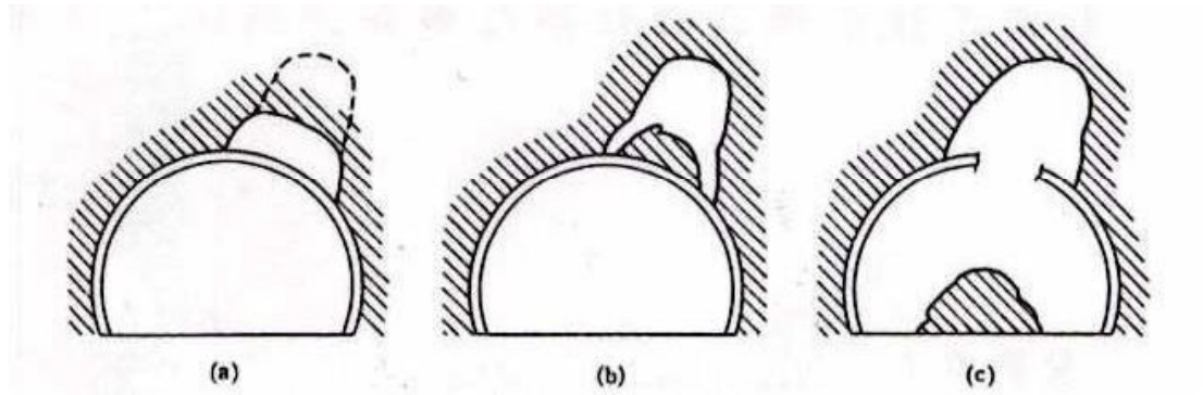
図 4 突発性崩壊の例
