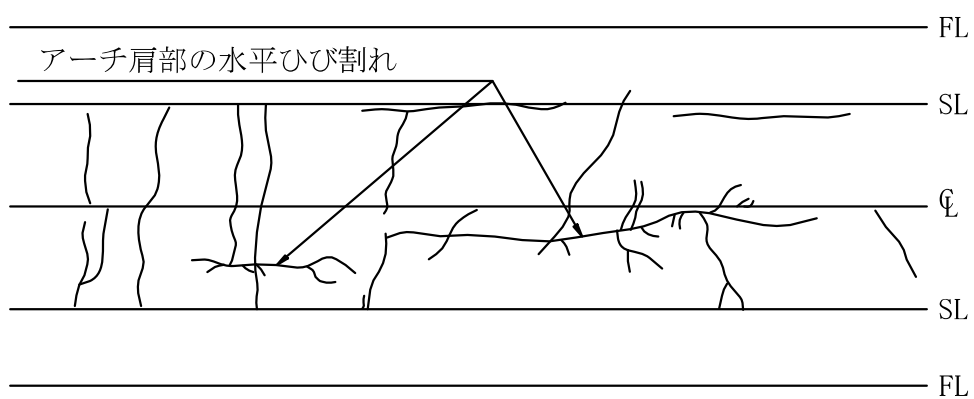
図7 偏土圧，斜面崩壊による変状の例
