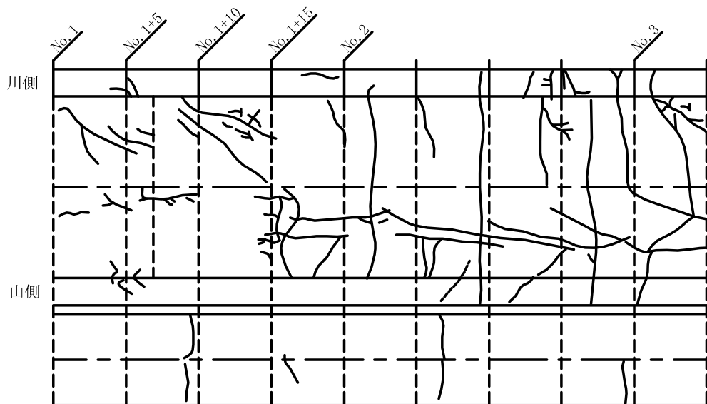
図 8 偏土圧と支持力不足の複合事例
