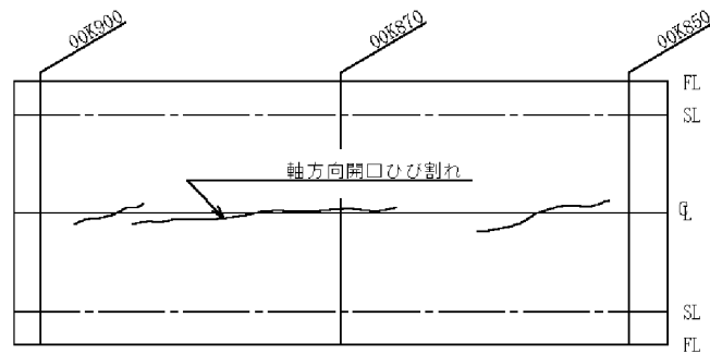
図1 緩み土圧の変状展開図の例
