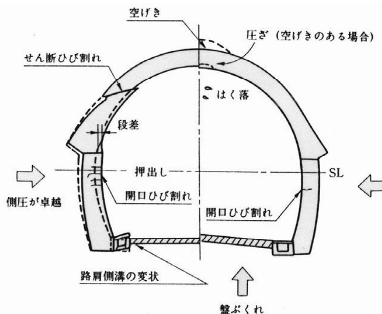
図 9 膨張性土圧による変状の模式図
