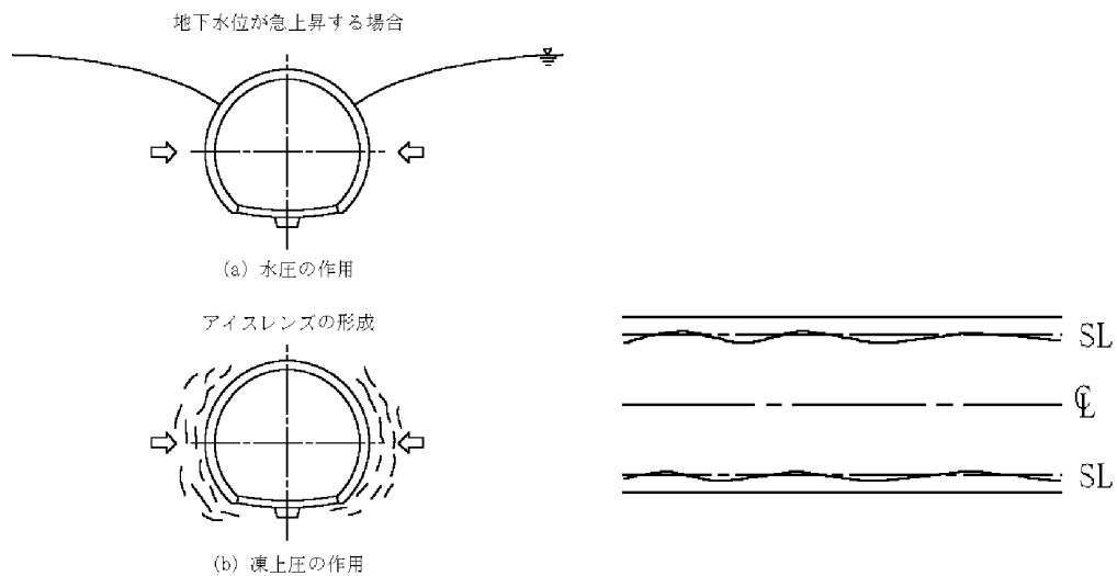
図 1 6 水圧・凍上圧
