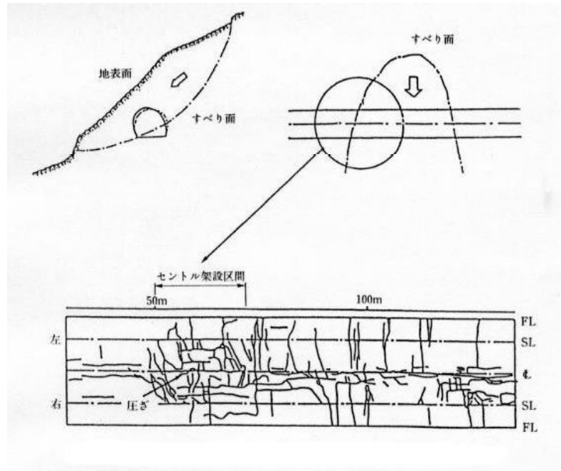
図 1 5 地すべり
