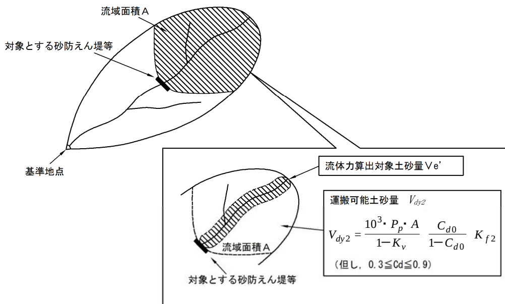
図Ⅲ- 4.7 土石流ピーク流量の算出
