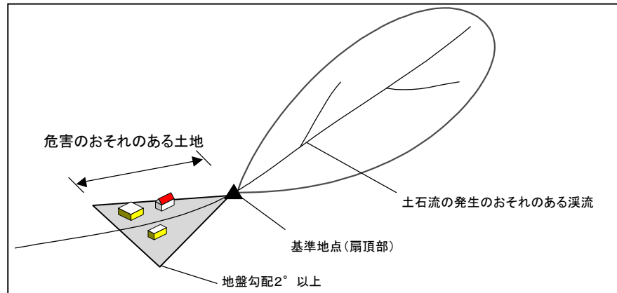
図III- 1.1 調査対象箇所の概念図
