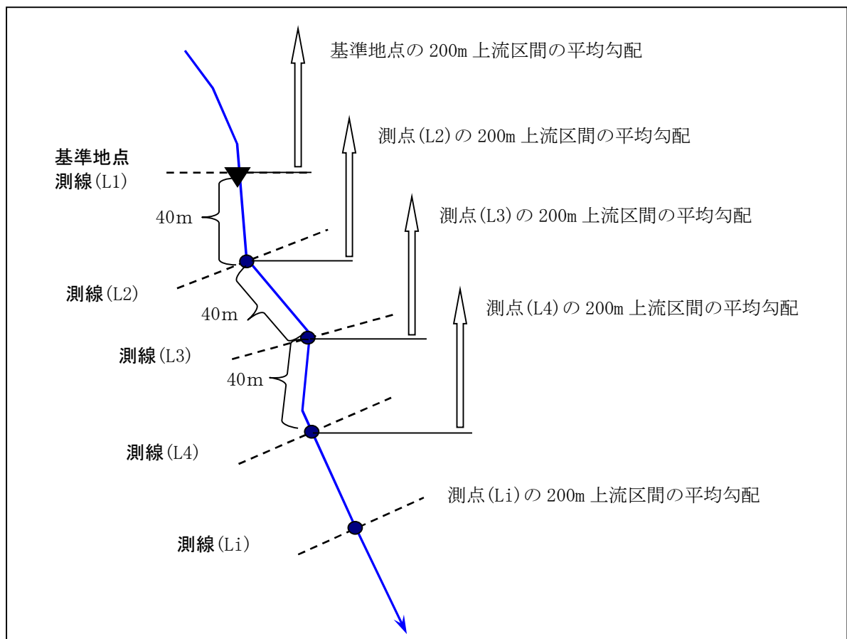
図Ⅲ- 6.9 区間勾配の設定イメージ
