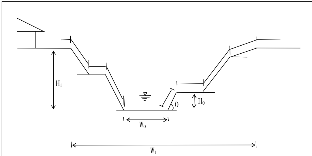
図III- 2.20 横断形状計測のイメージ図
