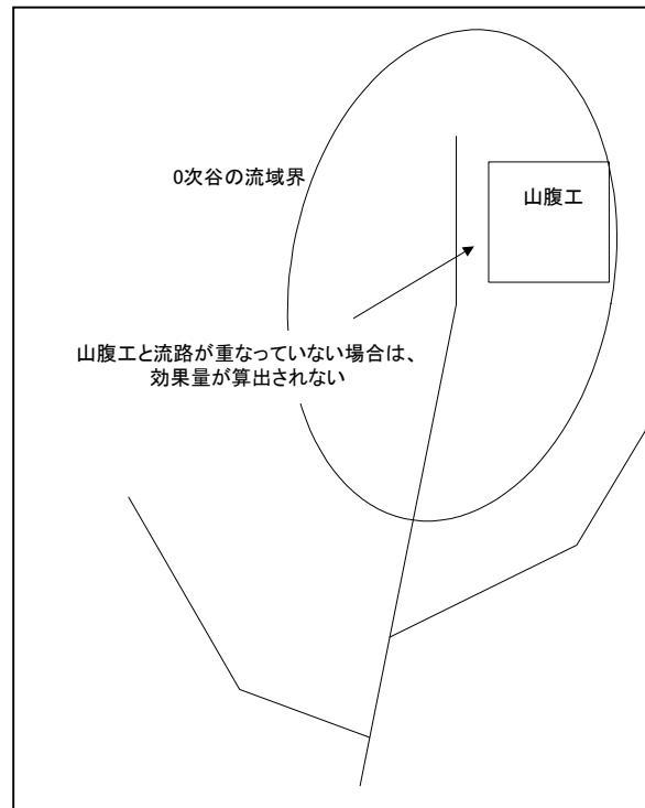
図Ⅲ- 4.4 山腹工の効果が見込めない例
